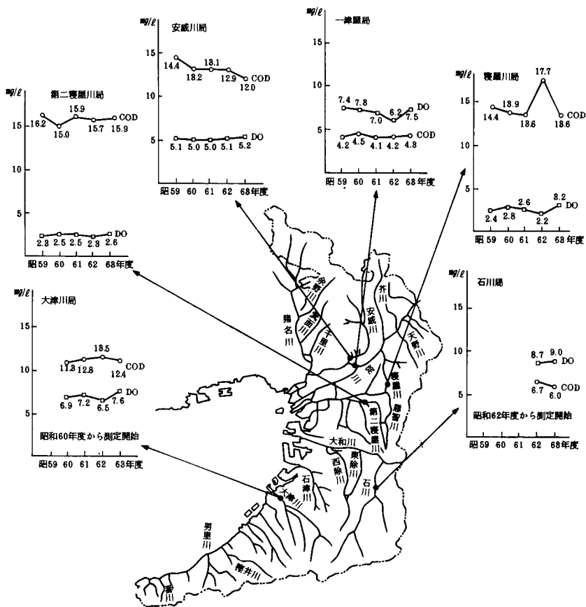
図2-3-9 COD、DO濃度（年平均値）の推移
