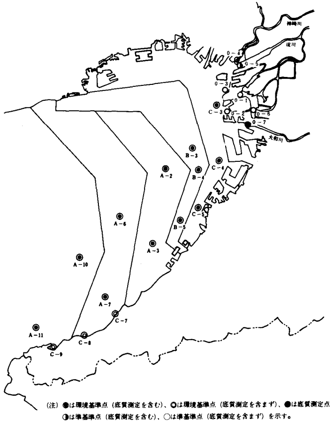
図2-3-10 大阪湾の測定地点図（昭和63年度）
