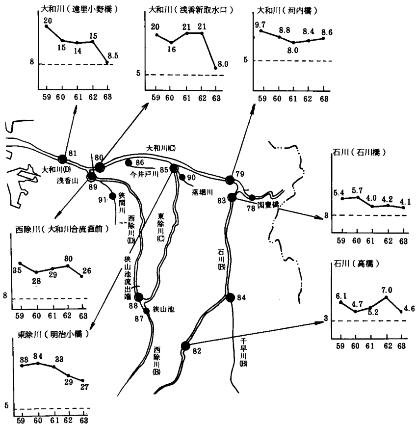
図2-3-7 大和川流域の水質測定地点及びBOD年平均値の推移
