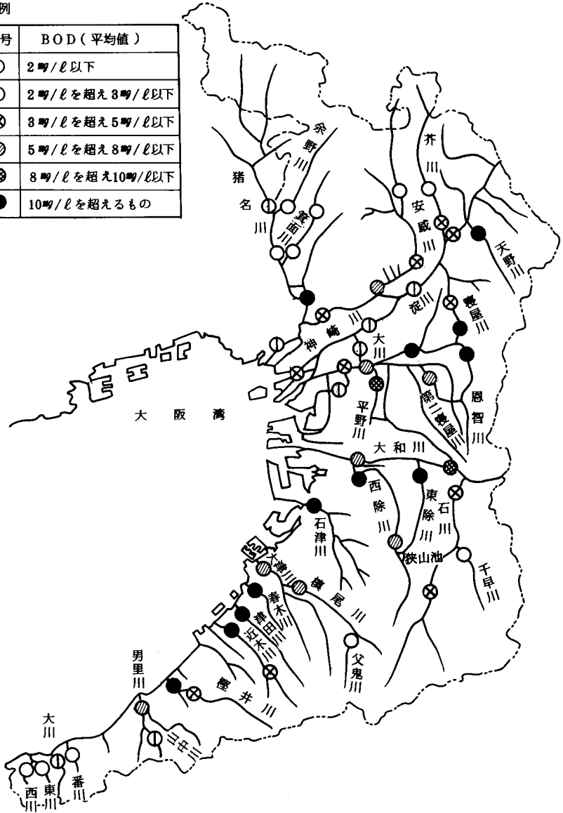
図2-3-2 府下の河川の水質（BOD）の概況（昭和63年度）
