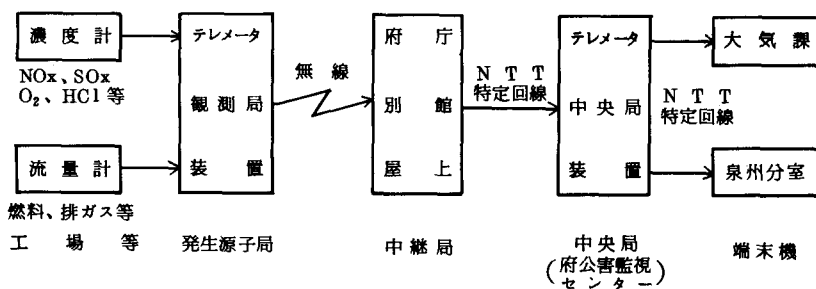
図 2-2-20 大気汚染発生源常時監視システム
