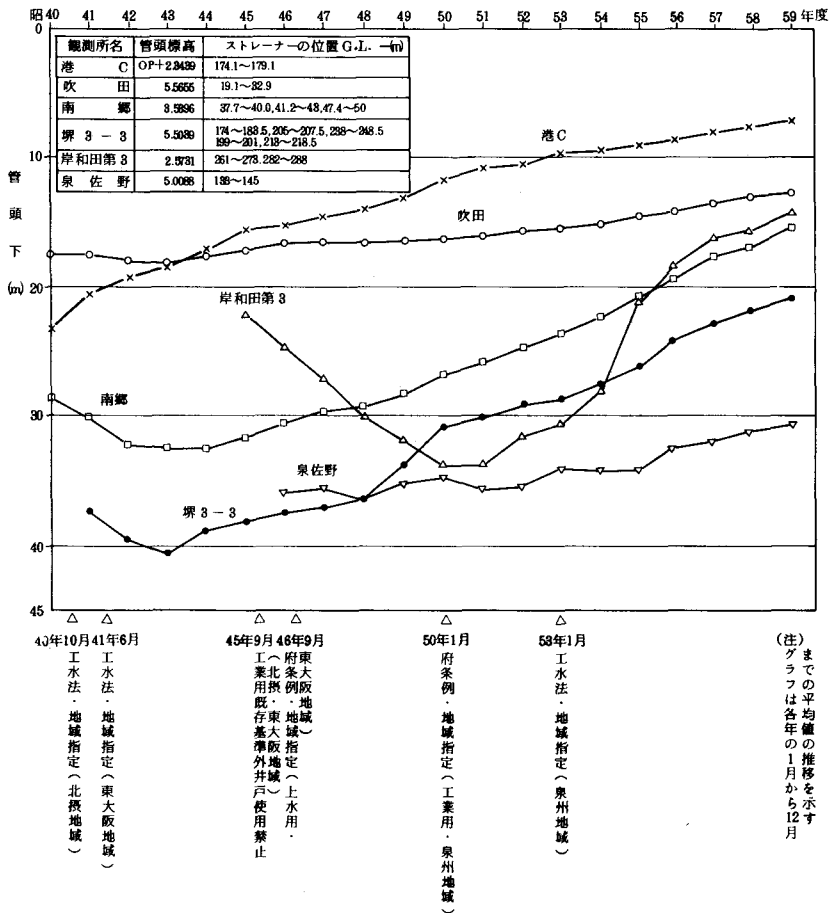
図2-7-2 地下水位の推移
