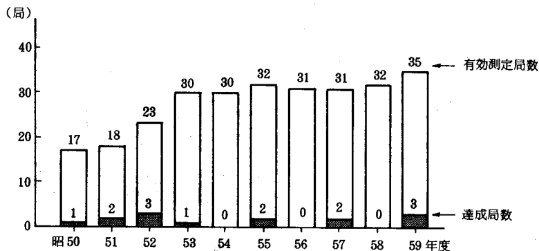
図 2-2-8 浮遊粒子状物質濃度の環境基準達成状況 (長期的評価)の推移
