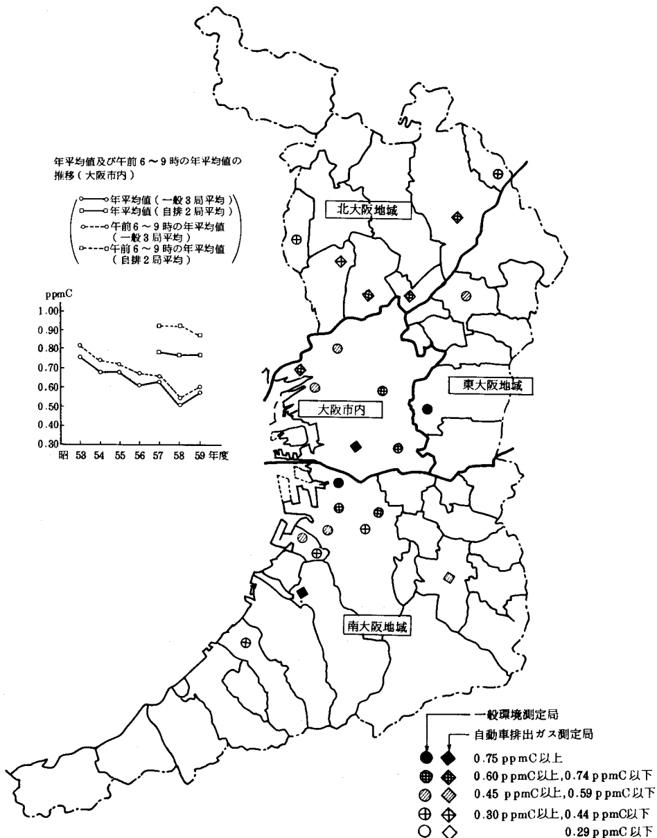
図 2-2-12 非メタン炭化水素濃度(年平均値)の概要(昭和59年度) と推移(年平均値及び午前6~9時の年平均値)
