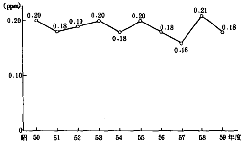
図2-2-17 光化学オキシダント濃度最高値（1時間値）の推移
