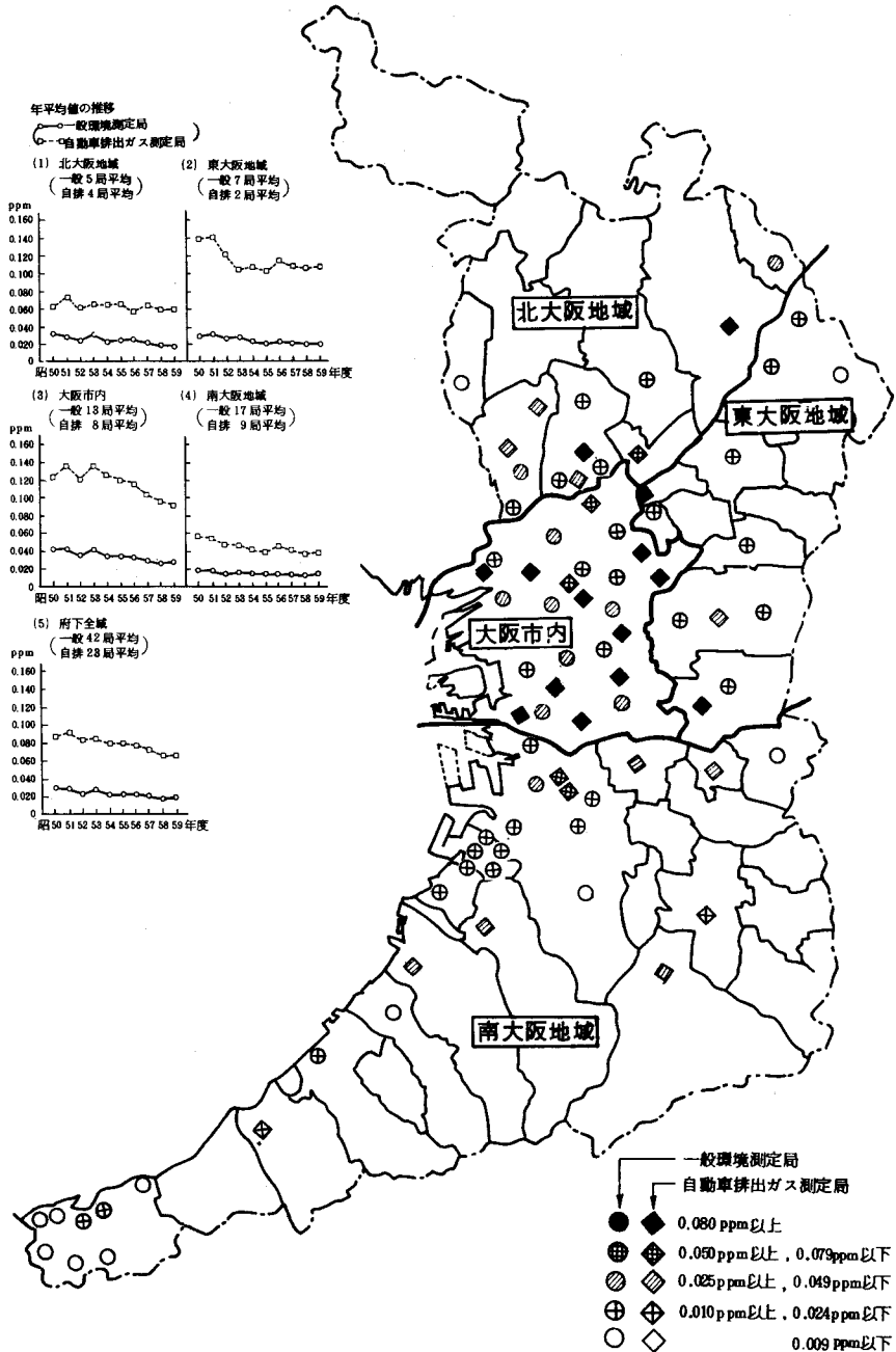
図 2-2-6 一酸化窒素濃度（年平均値）の概要（昭和 59 年度）と推移
