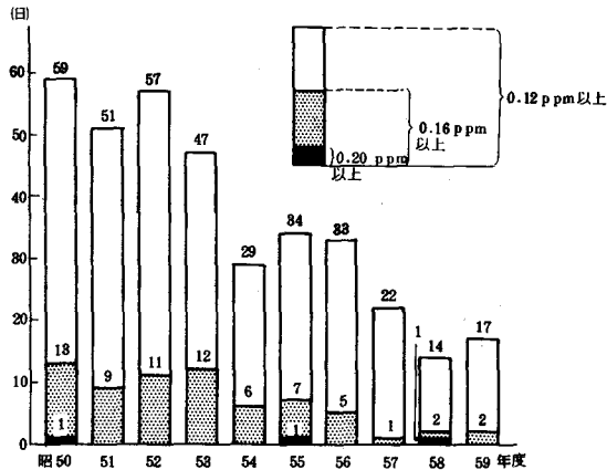
図2-2-18 光化学オキシダントが高濃度になった日数の推移（4～10月について基準測定点で集計）
