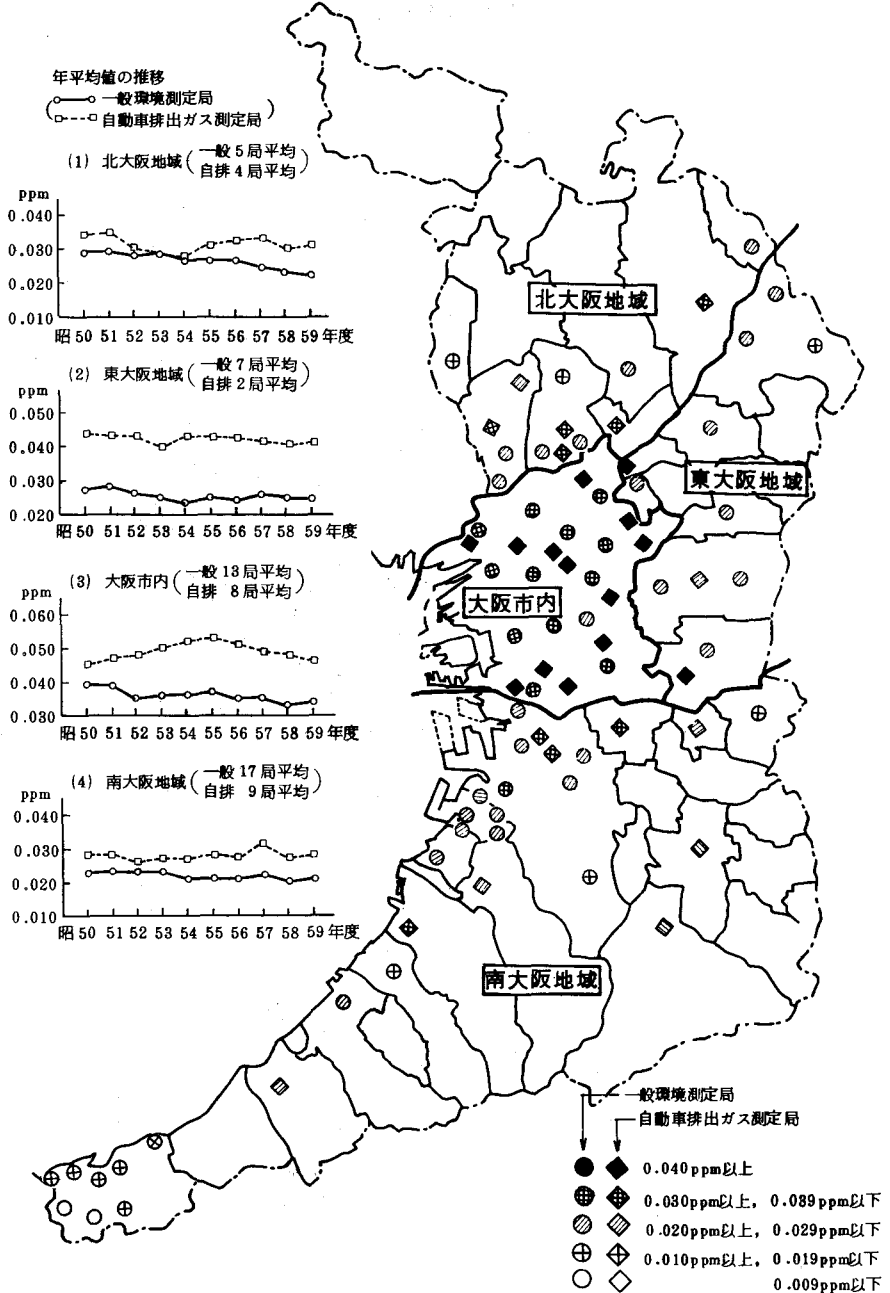
図 2-2-3 二酸化窒素濃度（年平均値）の概要（昭和59年度）と推移
