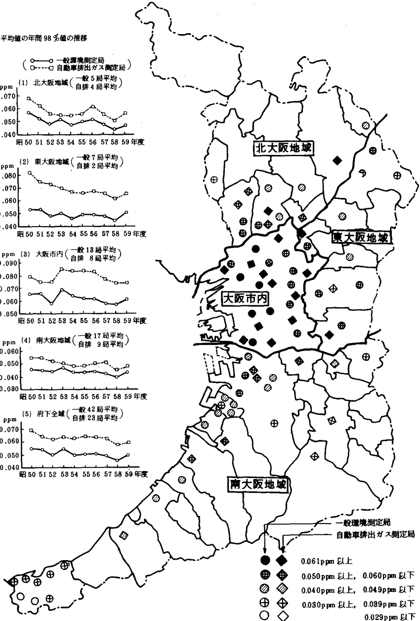
図2-2-4 二酸化窒素濃度（日平均値の年間98％値）の概要（昭和59年度）と推移
