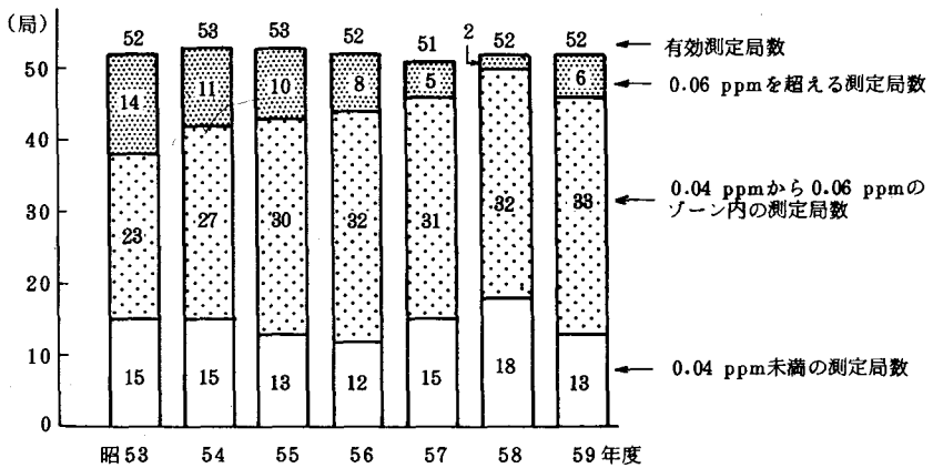
図2-2-5 二酸化窒素の環境基準達成状況の推移
