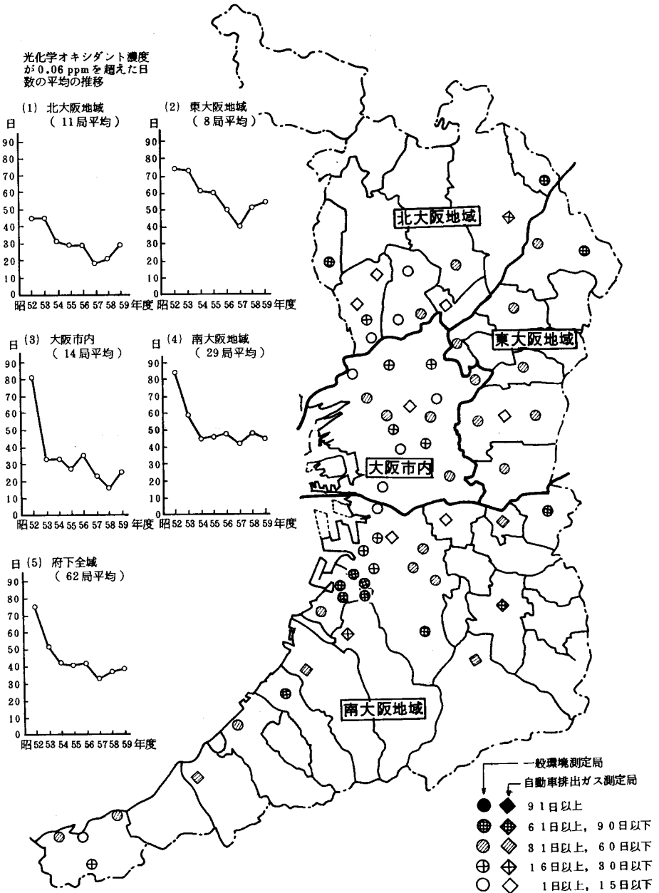
図2-2-15 光化学オキシダント濃度が0.06ppmを超えた日数の概要(昭和59年度)と推移
