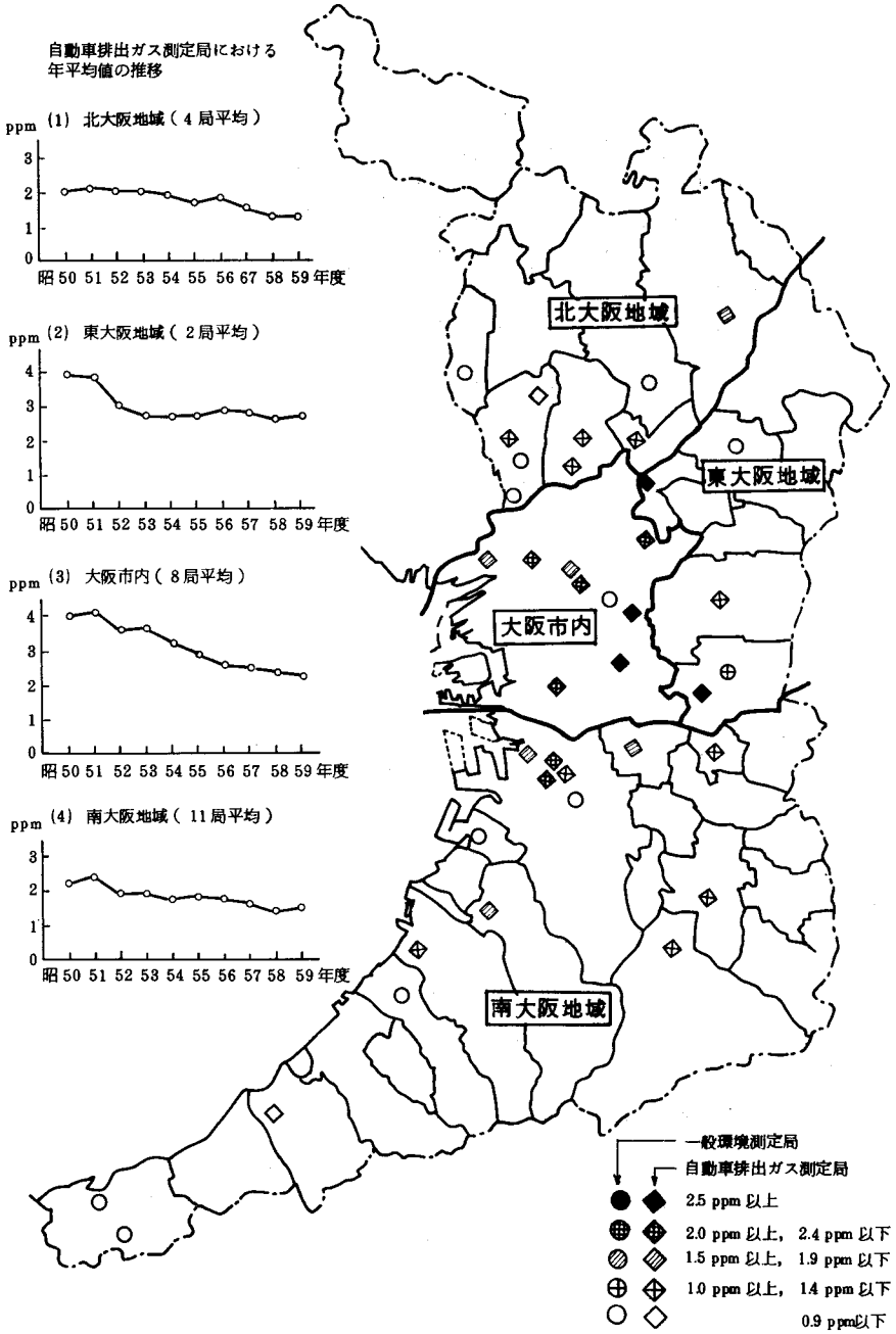
図 2-2-10 一酸化炭素濃度(年平均値)の概要(昭和 59 年度)と推移
