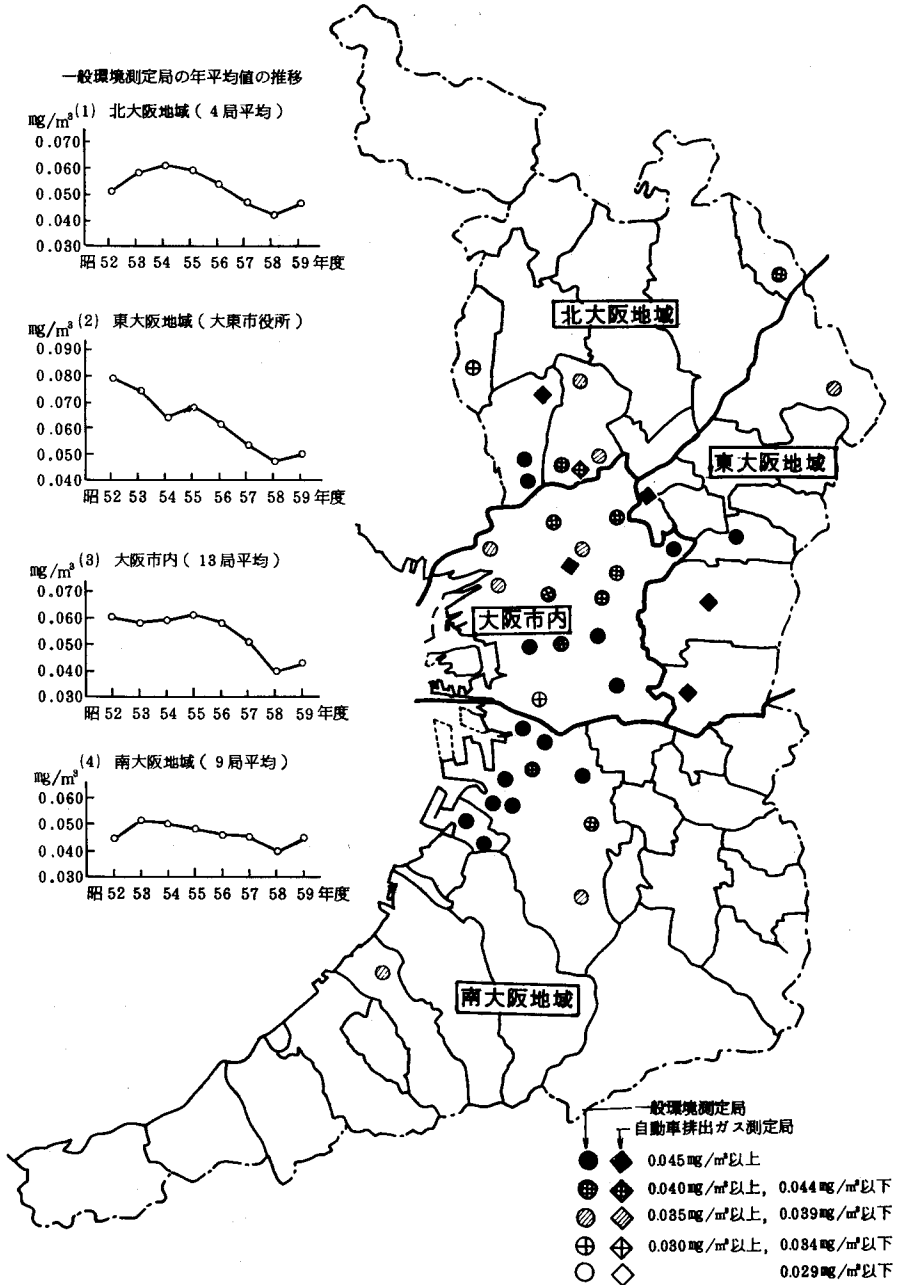
図 2-2-7 浮遊粒子状物質濃度(年平均値)の概要(昭和 59 年度)と推移
