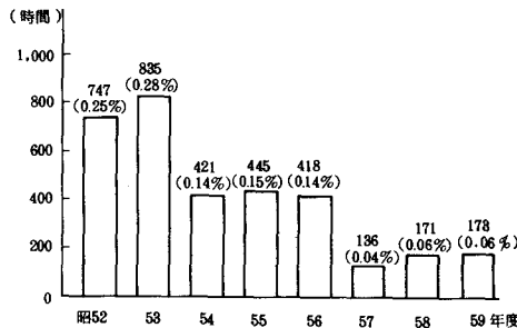
図 2-2-14 昼間の光化学オキシダント濃度が 0.12ppm 以上の総時間数の推移
