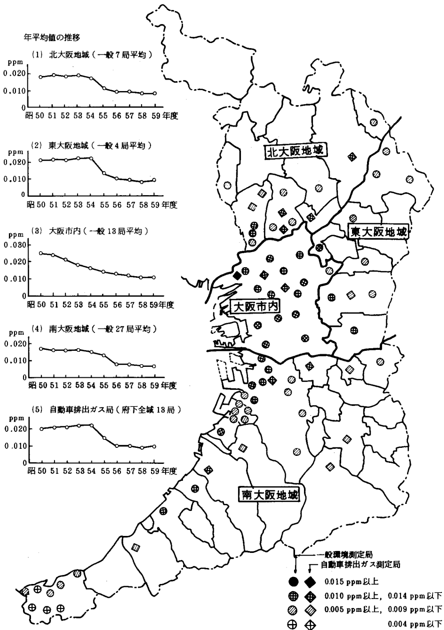
図 2-2-1 二酸化硫黄濃度(年平均値)の概要(昭和59年度)と推移
