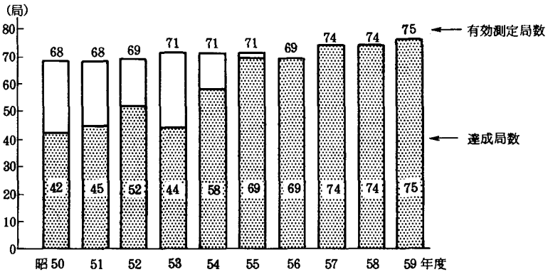
図 2 - 2 - 2 二酸化硫黄に係る環境基準達成状況（長期的評価）の推移
