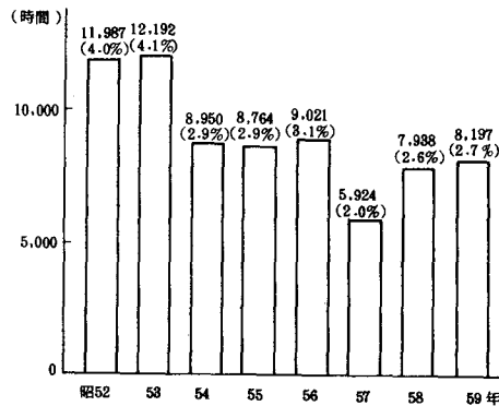
図 2-2-13 昼間の光化学オキシダント濃度が 0.06ppm を超えた総時間数の推移
