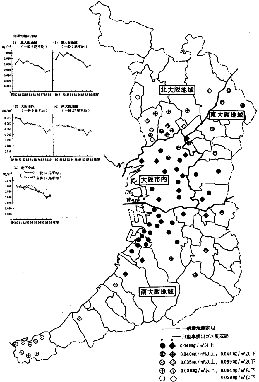
図 2-2-9 浮遊粉じん濃度（年平均値）の概要（昭和 59 年度）と推移
