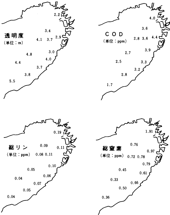
図2-2-14 大阪湾のCOD等の湾内分布(昭和53年度平均値)
