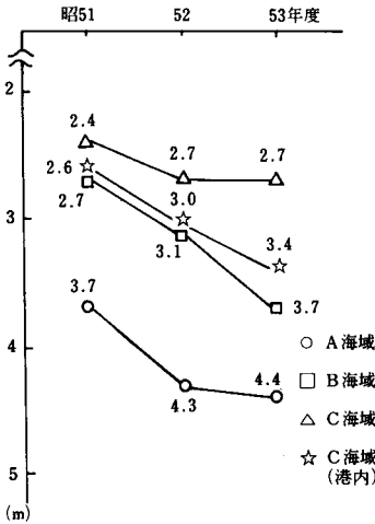
図2-2-12 大阪湾の透明度経年変化(年度平均値)
