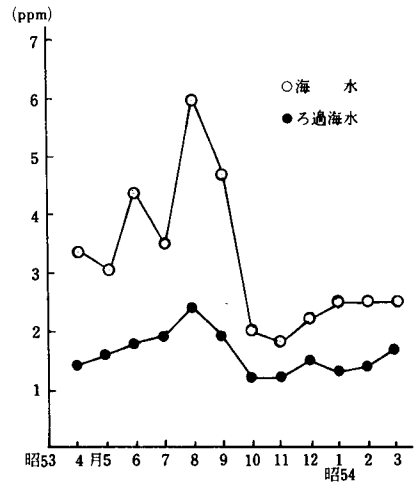
図2-2-13 大阪湾のCOD経月変化(昭和53年度) (港内3地点を除く12地点の平均)
