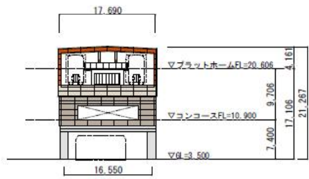
南側立面図
