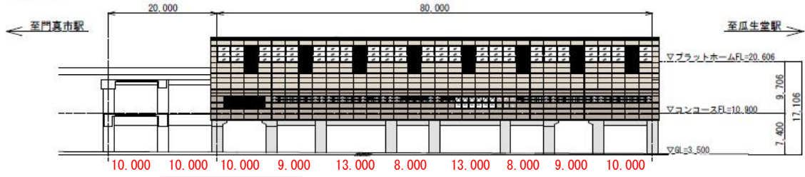
西側立面図
