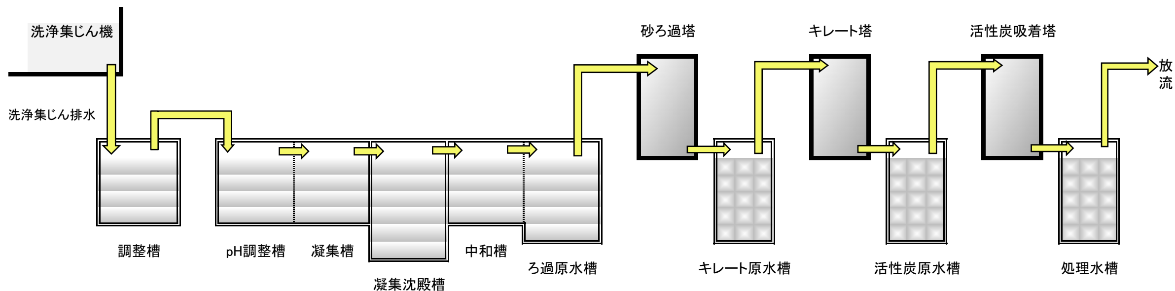
排水処理施設(洗浄集じん排水)の処理方式別
