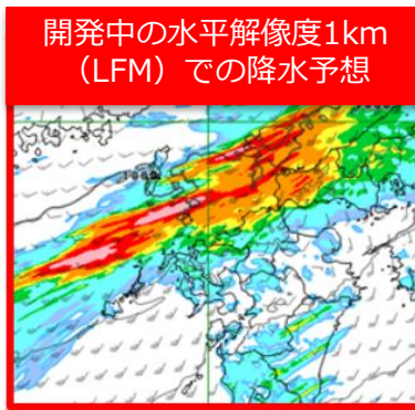
水平解像度1kmに高解像度化した局地モデルのイメージ
