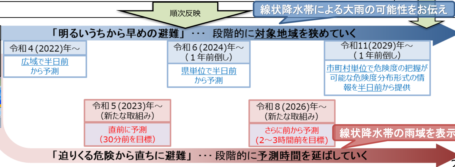
線状降水帯の雨域を楕円で表示
