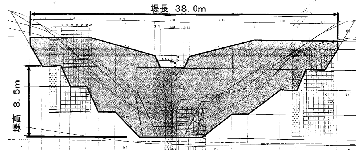
標準断面図
