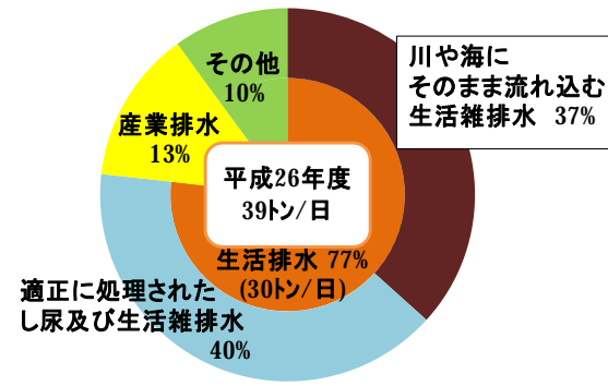
汚濁負荷量(BOD)の発生源別内訳(2014年度大阪府推計)
