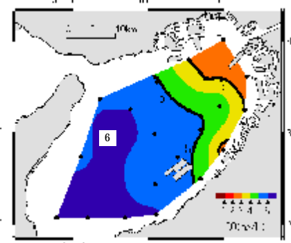
夏季底層DOの分布(2014～2016年度平均) 【出典】(地独)大阪府立環境農林水産総合研究所
