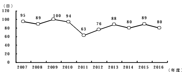
光化学オキシダントの屋間の濃度が 0.06ppm を超えた日数の推移
