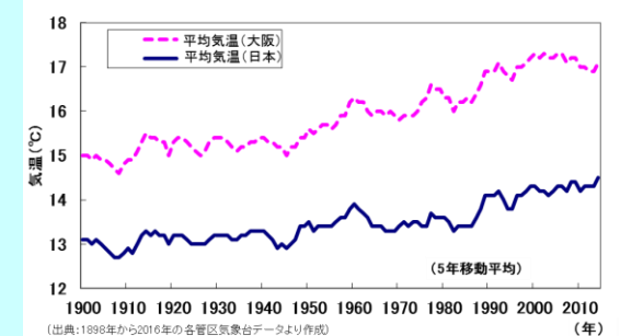
年平均気温の推移
