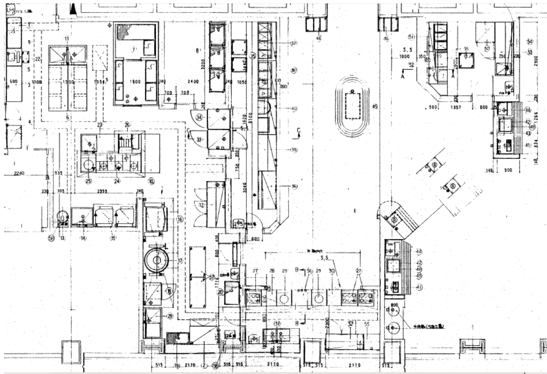
6階食堂平面図
