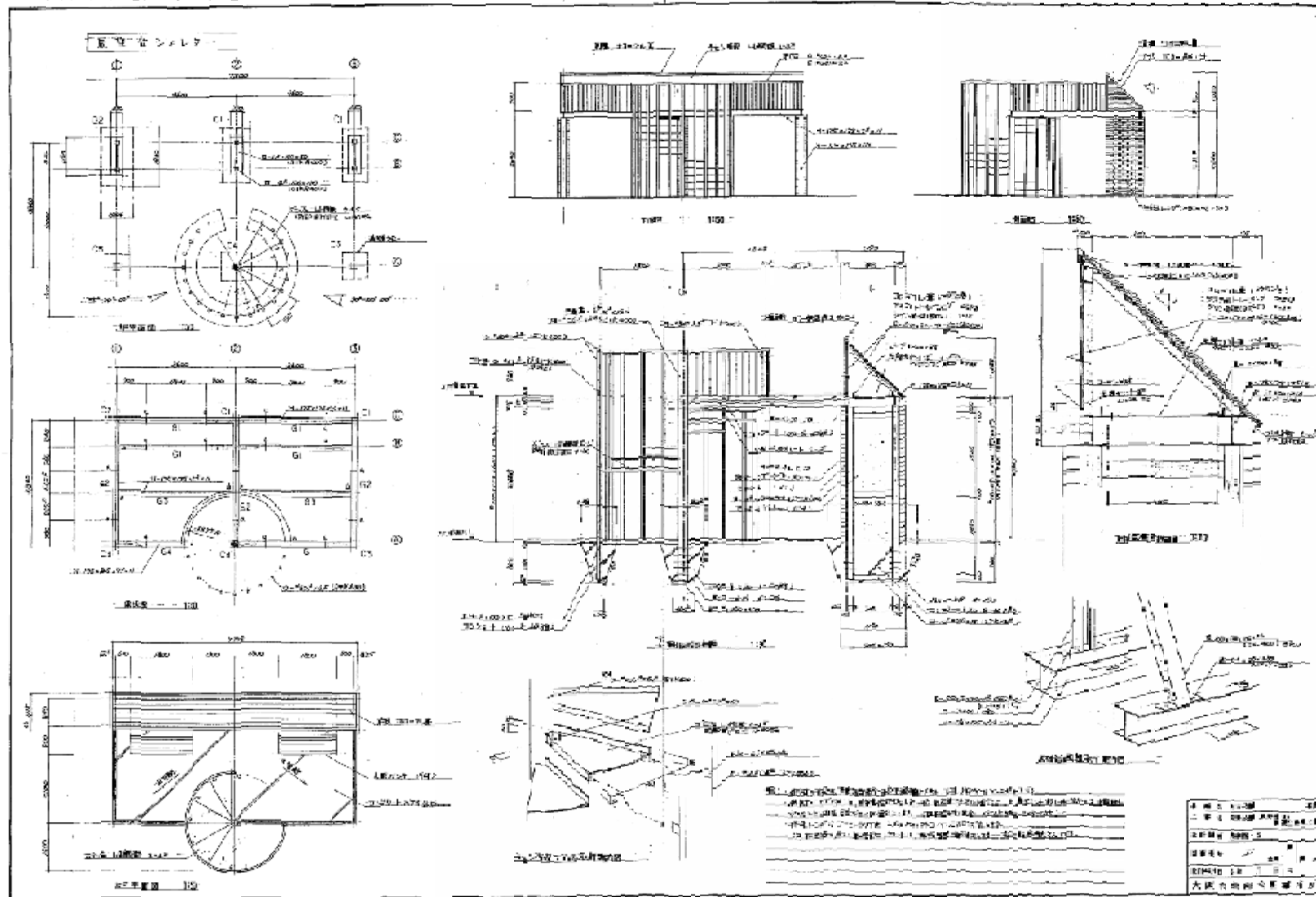
12-16 長野公園 主要建物図面（展望台）
