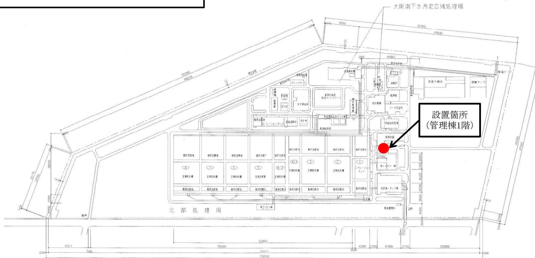
北部水みらいセンター平面図
