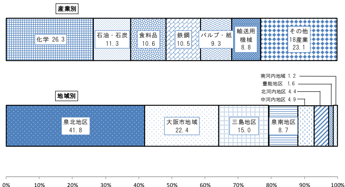
第35図 1日当たり用水総使用量の産業別・地域別構成比（従業者30人以上） （1日当たり用水総使用量 50万7,991m 3 ）
