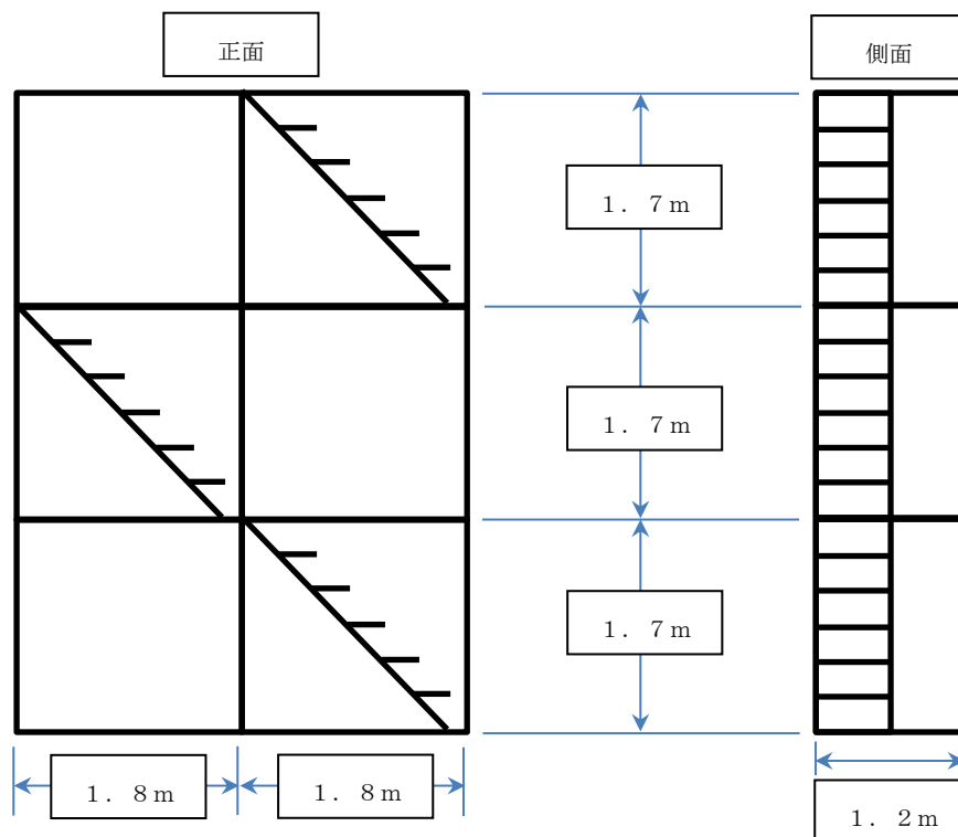
【写真撮影用枠組足場の設置例】
