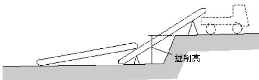
【 調査掘削時のベルトコンベヤ設置例 】
