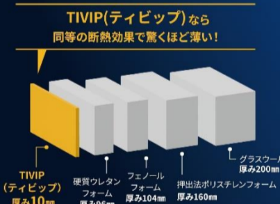
■断熱性能を同じにした時の各断熱材の厚みの違い
