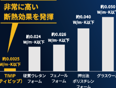
■各断熱材の熱伝導率の比較
