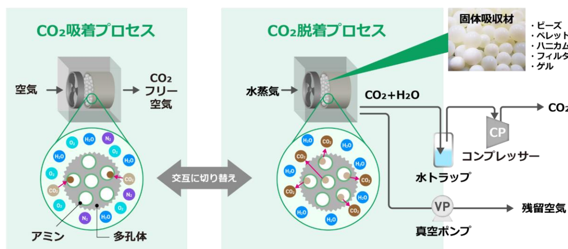
DACプロセスのイメージ
