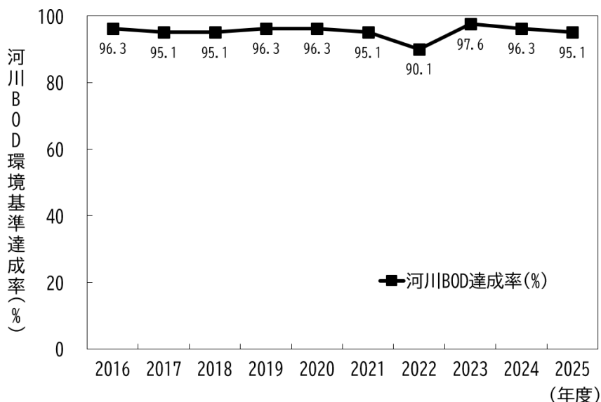
図2 河川のBOD環境基準達成率の推移
