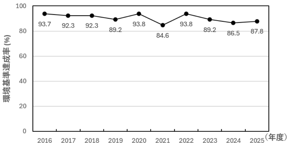
図4 河川的全亜鉛環境基準達成率の推移
