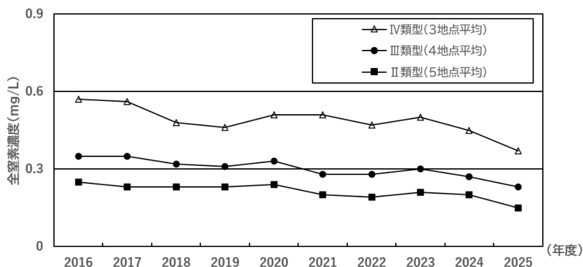
図 6 大阪湾の全窒素濃度（表層年平均値）の推移（大阪府測定地点）
