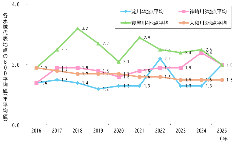
図3 主要河川のBOD濃度（年平均値）の推移
