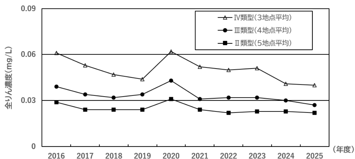
図7 大阪湾の全りん濃度（表層年平均値）の推移（大阪府測定地点）
