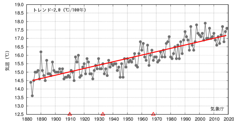
大阪 年平均気温1883-2019年
