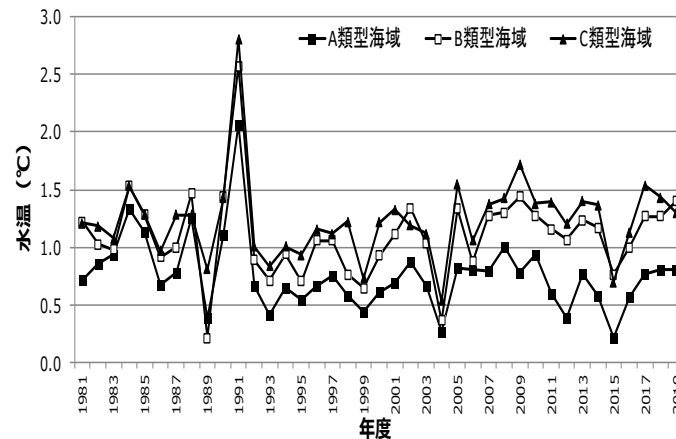
大阪湾における大阪府が測定する環境基準点 の表層と底層の水溫差の推移 (年平均: 湾東部12地点)
