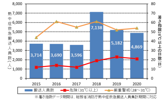
府域における熱中症による 救急搬送人員数と暑さ指数28℃以上の日数の推移
