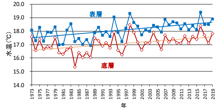
大阪湾の漁場環境の把握を目的とした 大阪湾全域の水温の推移(年平均値;20地点)
