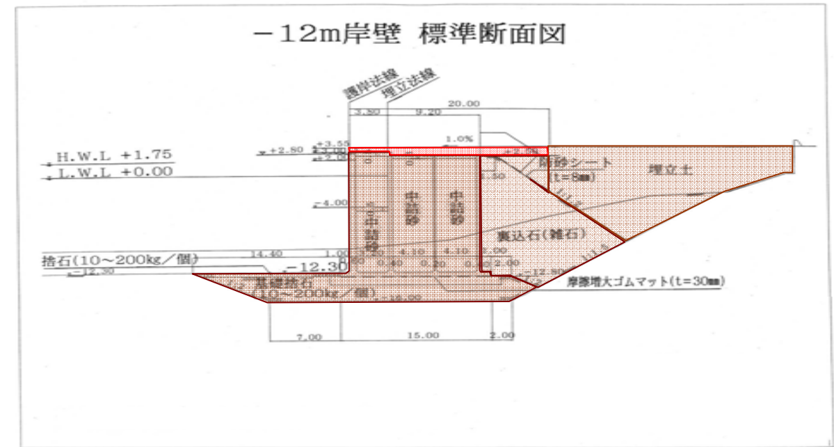
標準断面図
