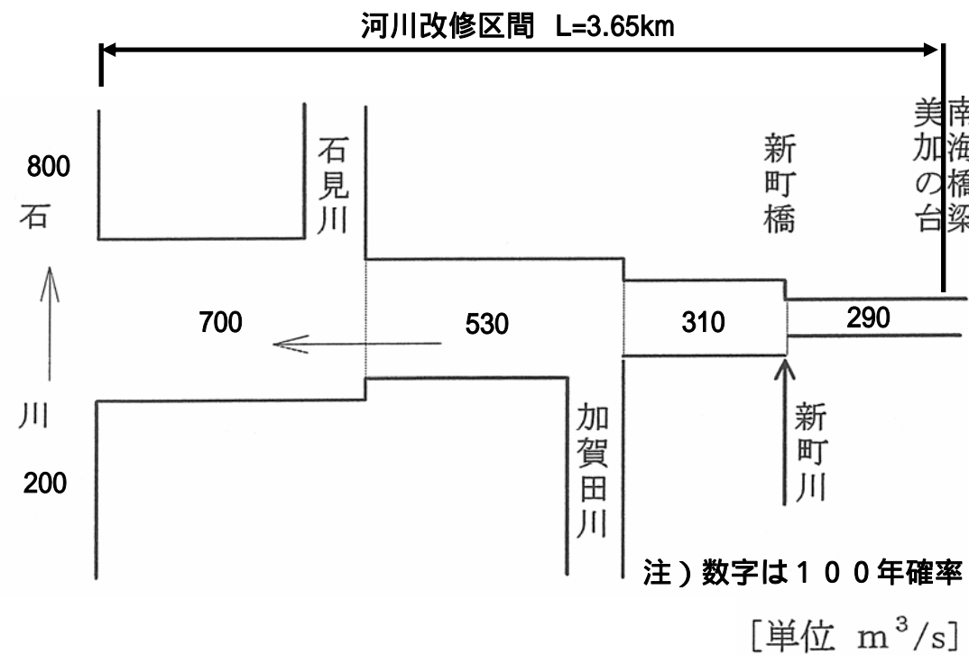
流量配分図
