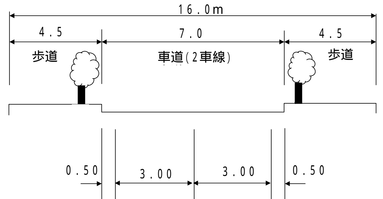
標準断面図
