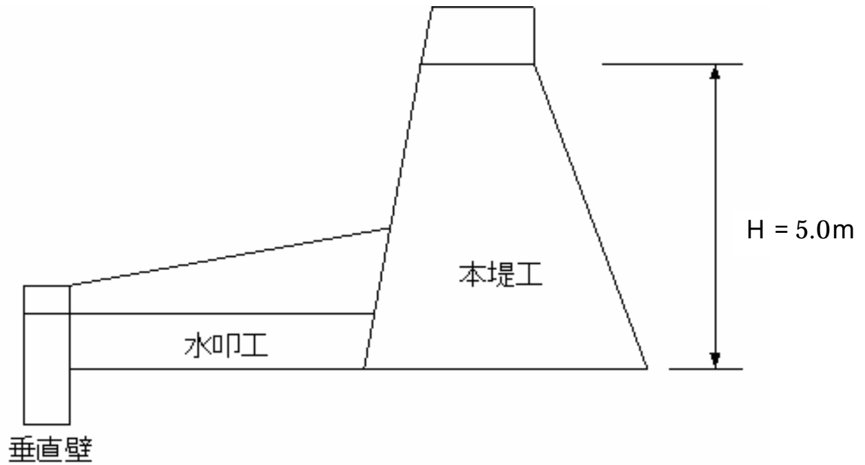
標準断面図
