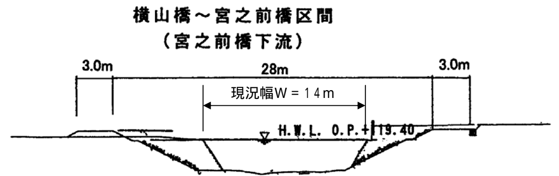
標準断面図
