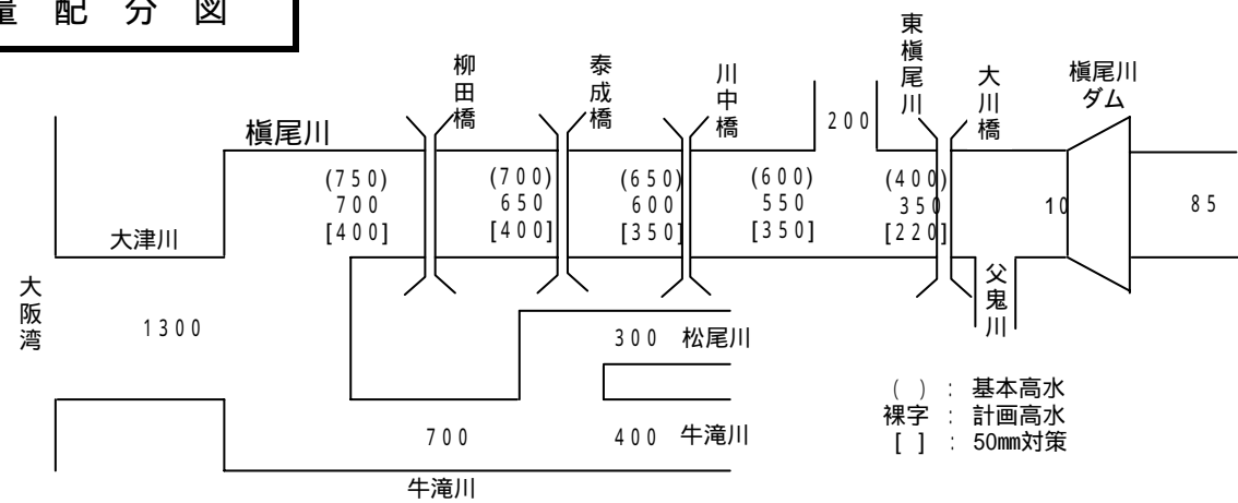
流量配分図
