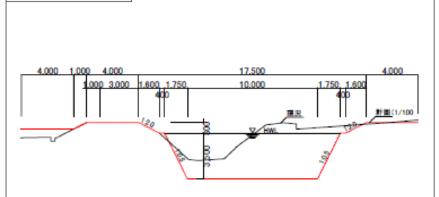
標準断面図
