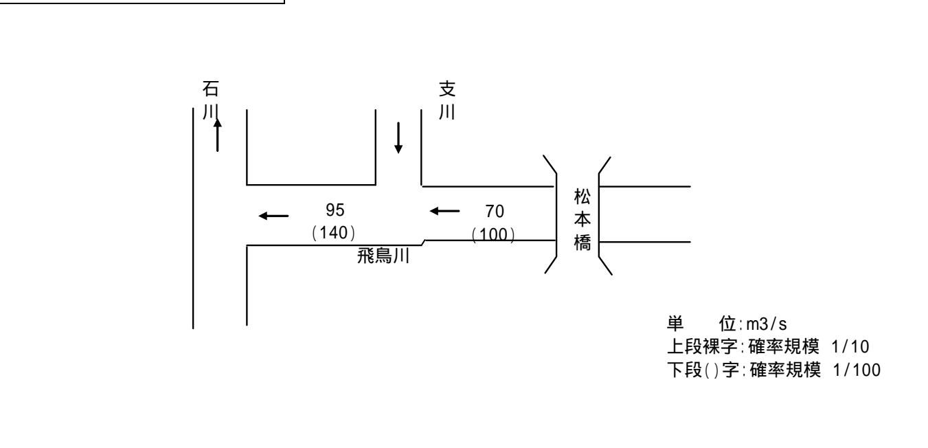
流量配分図
