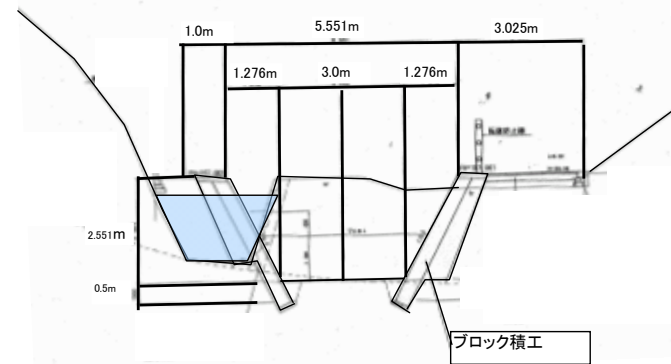
標準断面図
