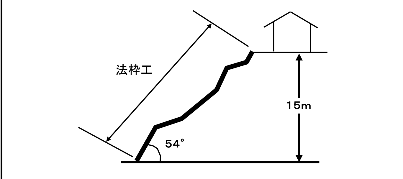
標準断面図
