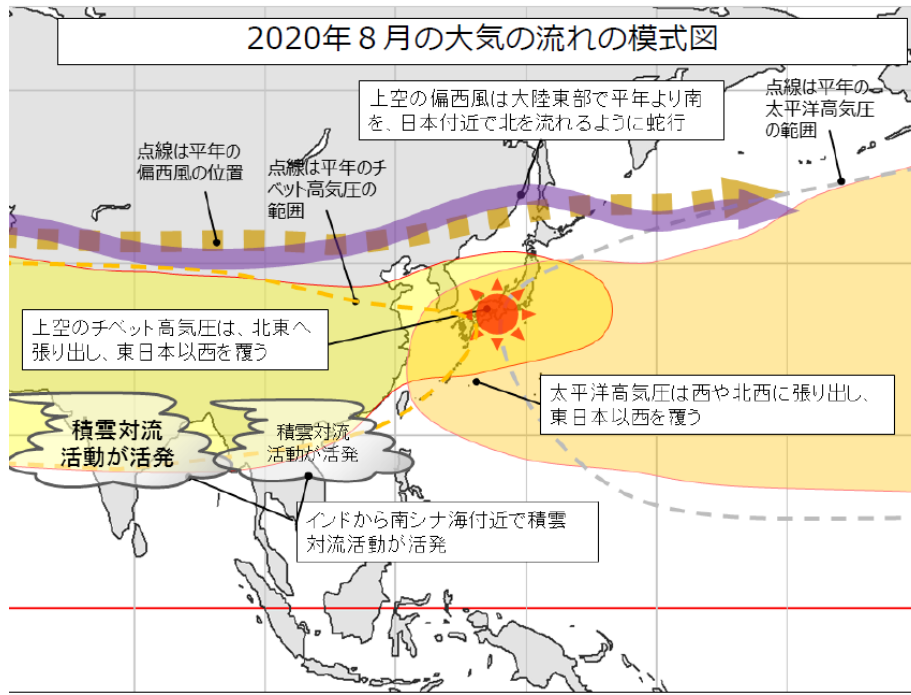
図1-2-3 2020年8月の大気の流れの模式図
