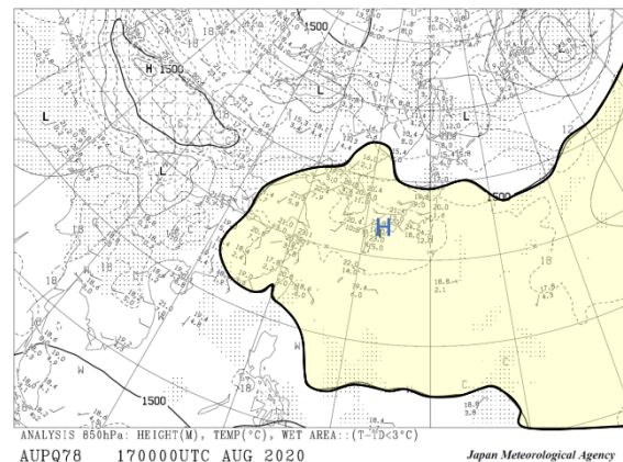
図1-2-5 8月17日09時 850hPa 天気図
