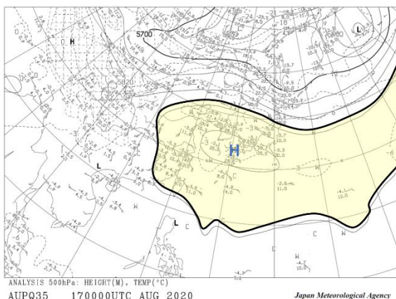
図1-2-4 8月17日09時 500hPa 天気図
