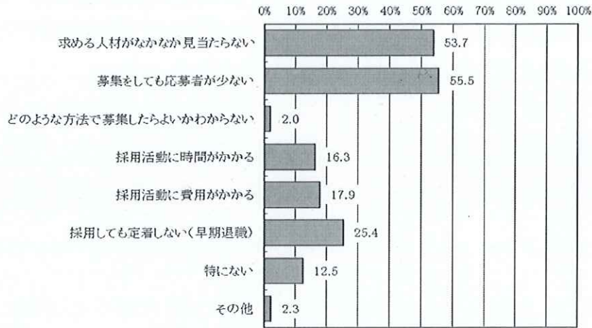
図7 若年労働者(34歳以下)を確保するうえでの課題
