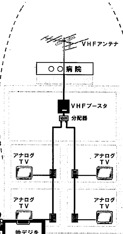
既存テレビ共聴設備
