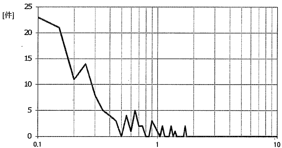
○建築物の解体等現場（集じん・排気装置排気口、総繊維数濃度）
