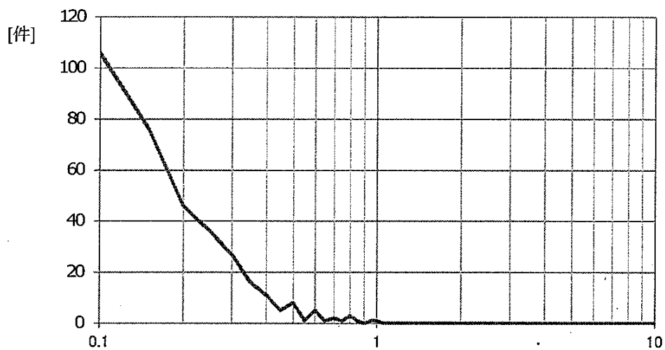
○建築物の解体等現場（敷地境界等、総繊維数濃度）
