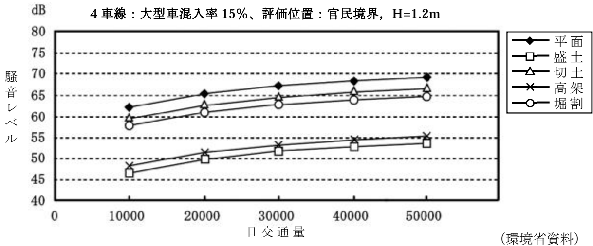
図5 交通量による夜間騒音レベルの変化
