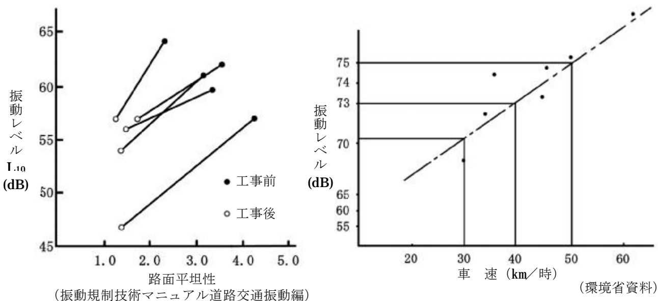
図9 修繕工事前後の振動レベルの関係例
