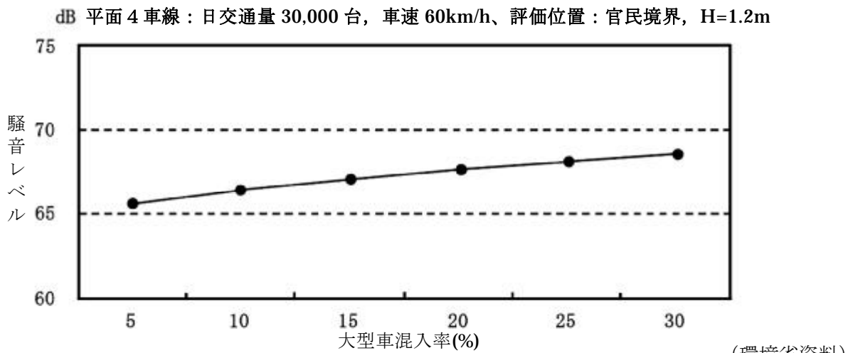
図6 大型車混入率による騒音レベルの変化
