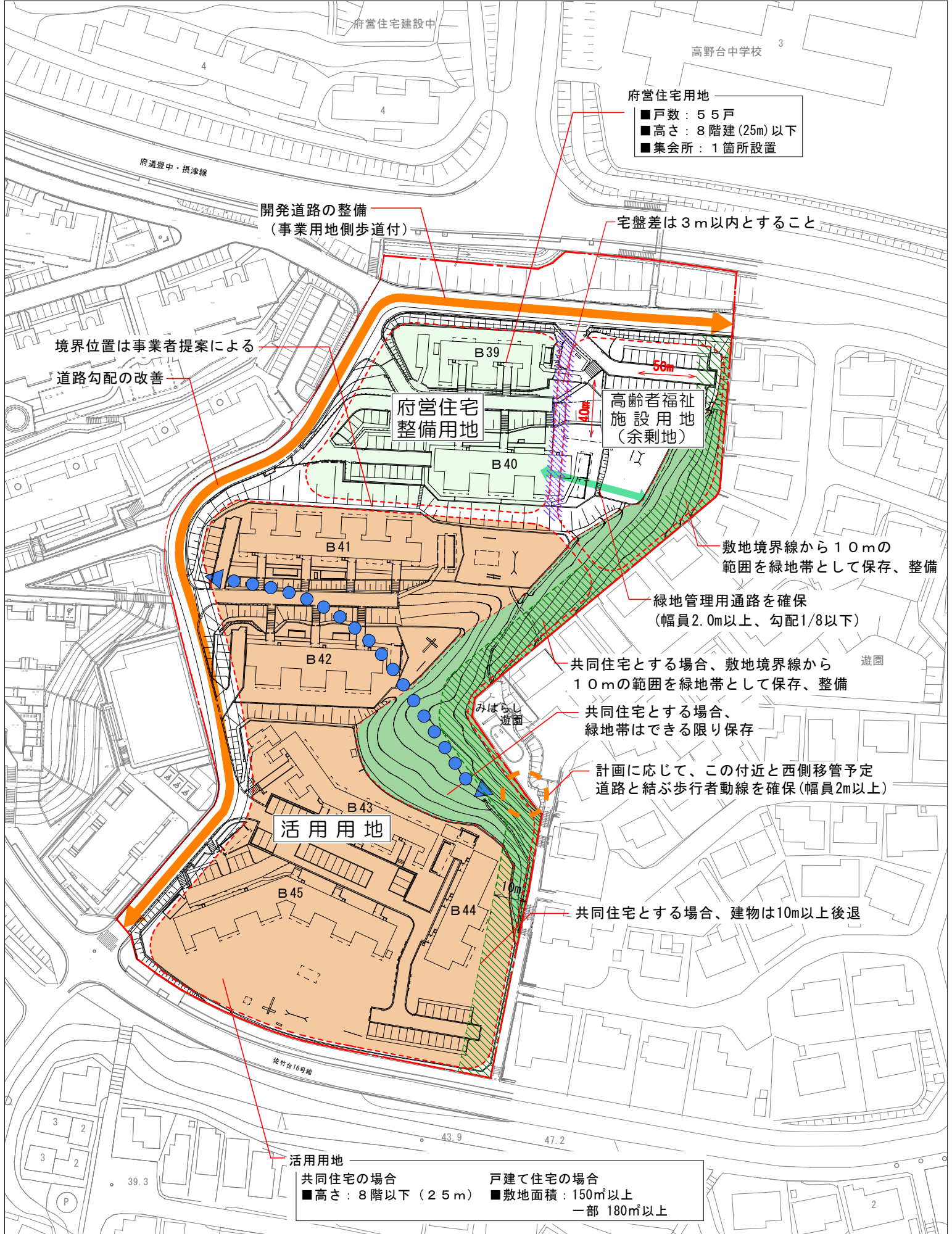
添付図4-1 吹田佐竹台住宅 土地利用計画図
