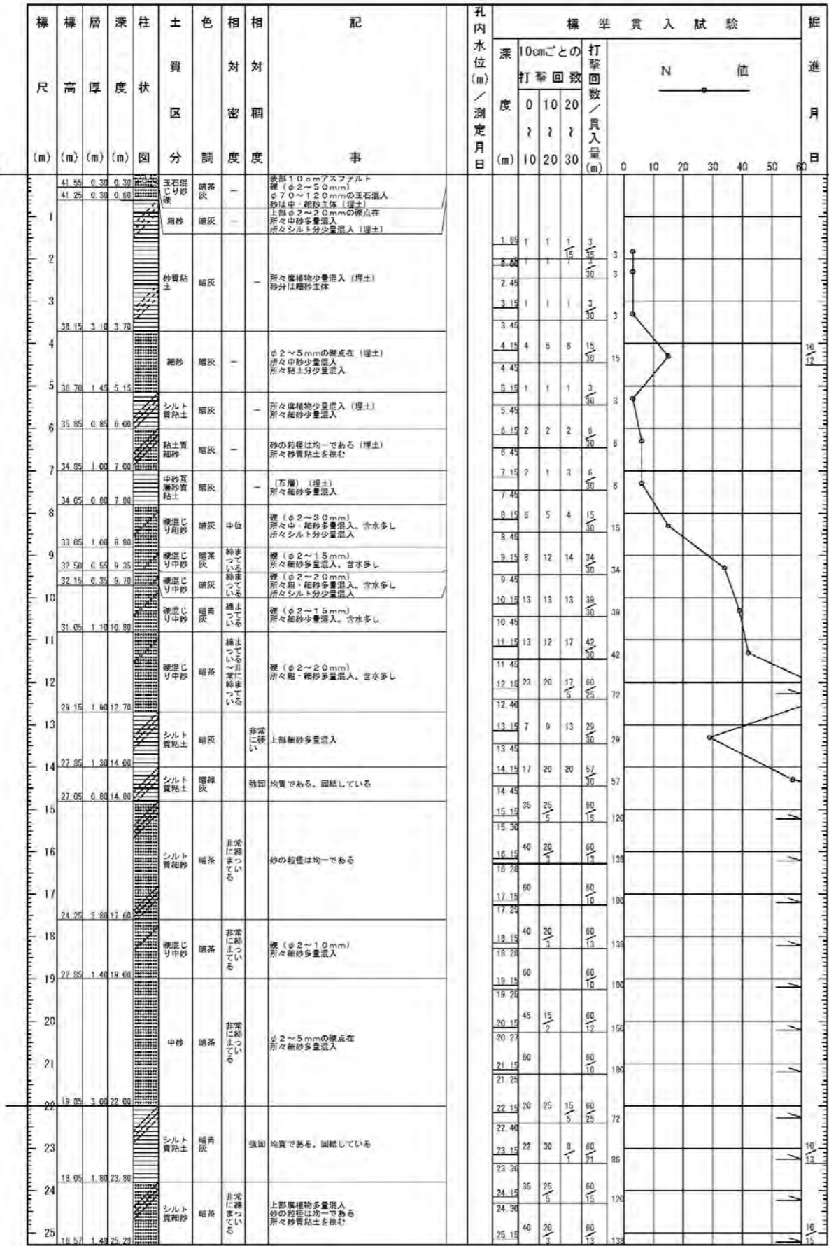
柱状図 D-1
