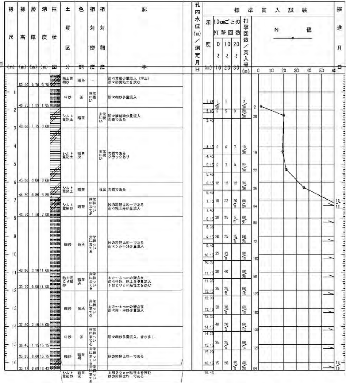
柱状図 E-1
