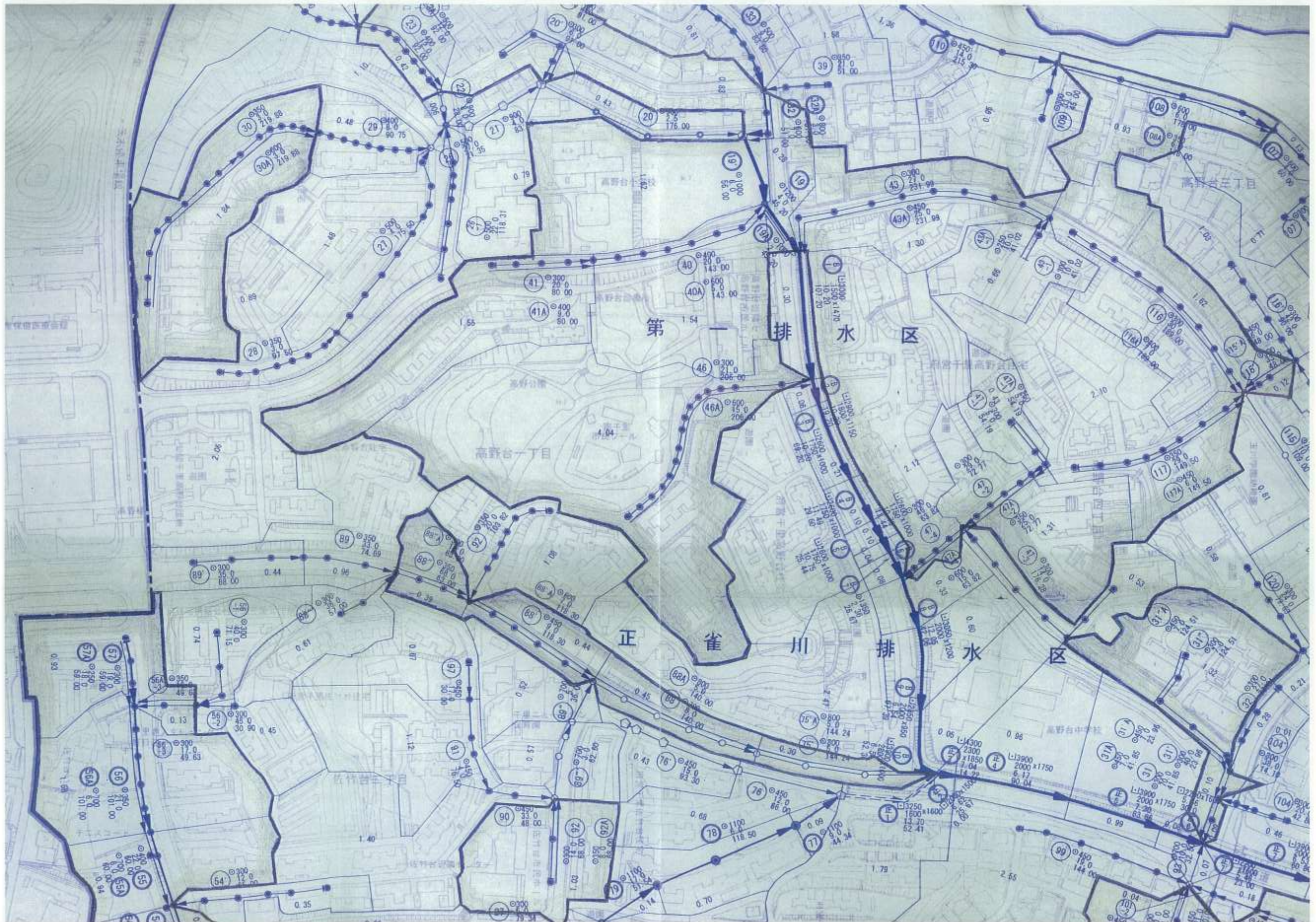
添付図 1 4 - 吹田市下水道計画 (雨水) (部分)
