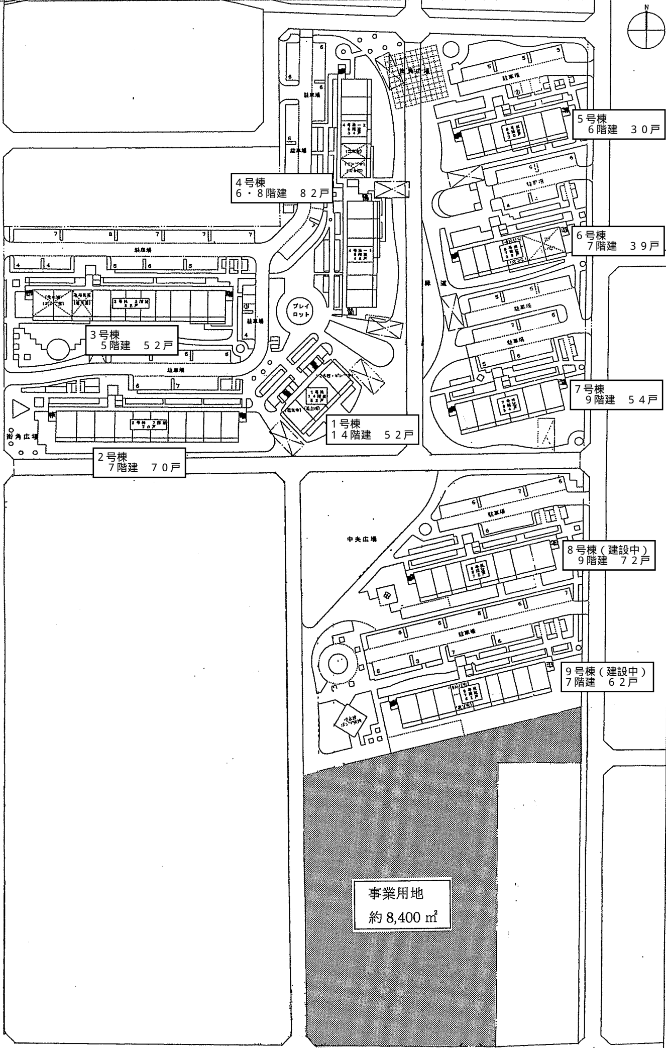
敷地図 (島之内住宅計画図)
