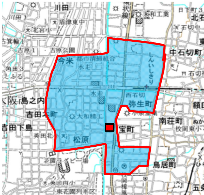
宝町調節池 集水区域図
