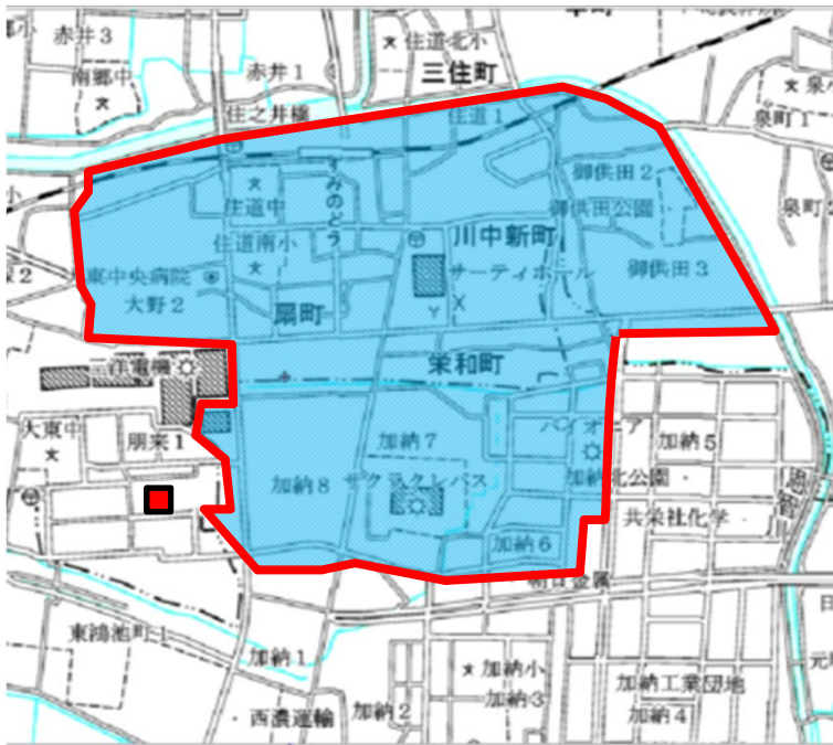
朋来調節池 集水区域図
