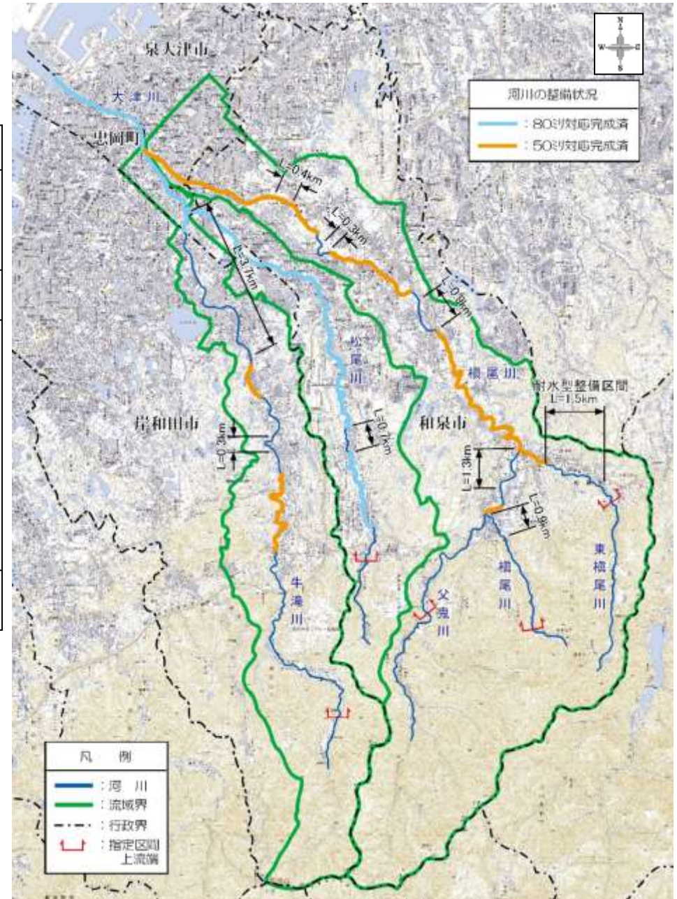
整備対象区間平面図（洪水対策）
