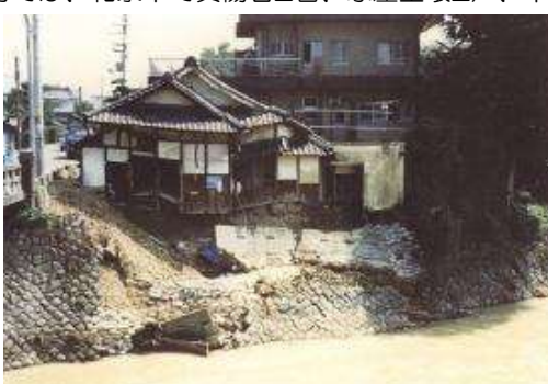
槇尾川川中橋下流（和泉市三林町）
