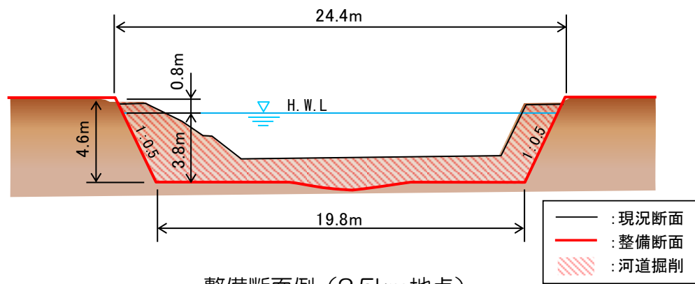
整備断面例（2.5km地点）
