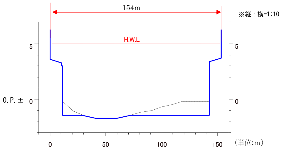
図 - 2.4 整備断面例 (神洲橋 かみす ～三国橋)
