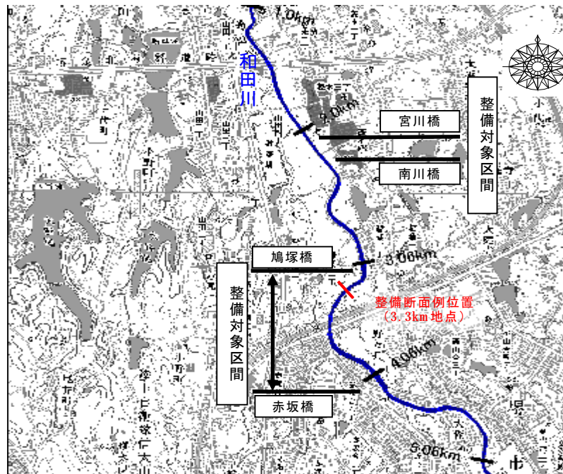
図 2.4 整備対象区間平面図
