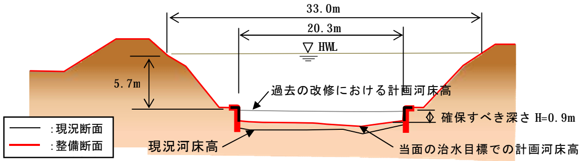
図 2.3 整備断面例 (3.9km地点)
