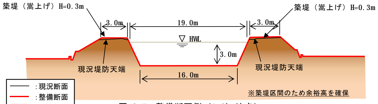
図 2.5 整備断面例 (1.9km地点)
