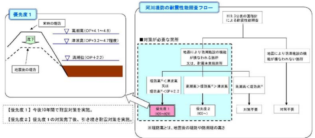
図 1.2.6 河川堤防の耐震性能照査フロー図
