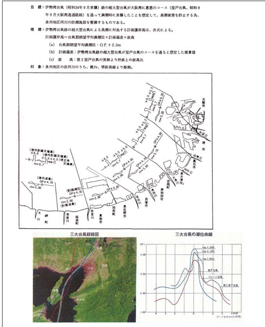
図 1.2.4 泉州河川高潮対策事業計画
