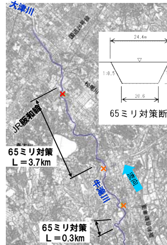
図 1.4.7 牛滝川の当面の治水目標の設定
