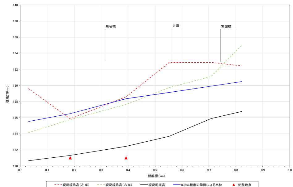
図 1.4.11 父尾川水位縦断面図（現況河道：時間雨量 65 ㎥程度）
