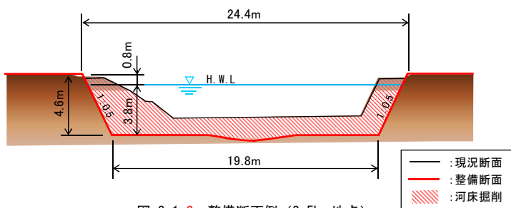
図 2.1.3 整備断面例 (2.5km 地点)
