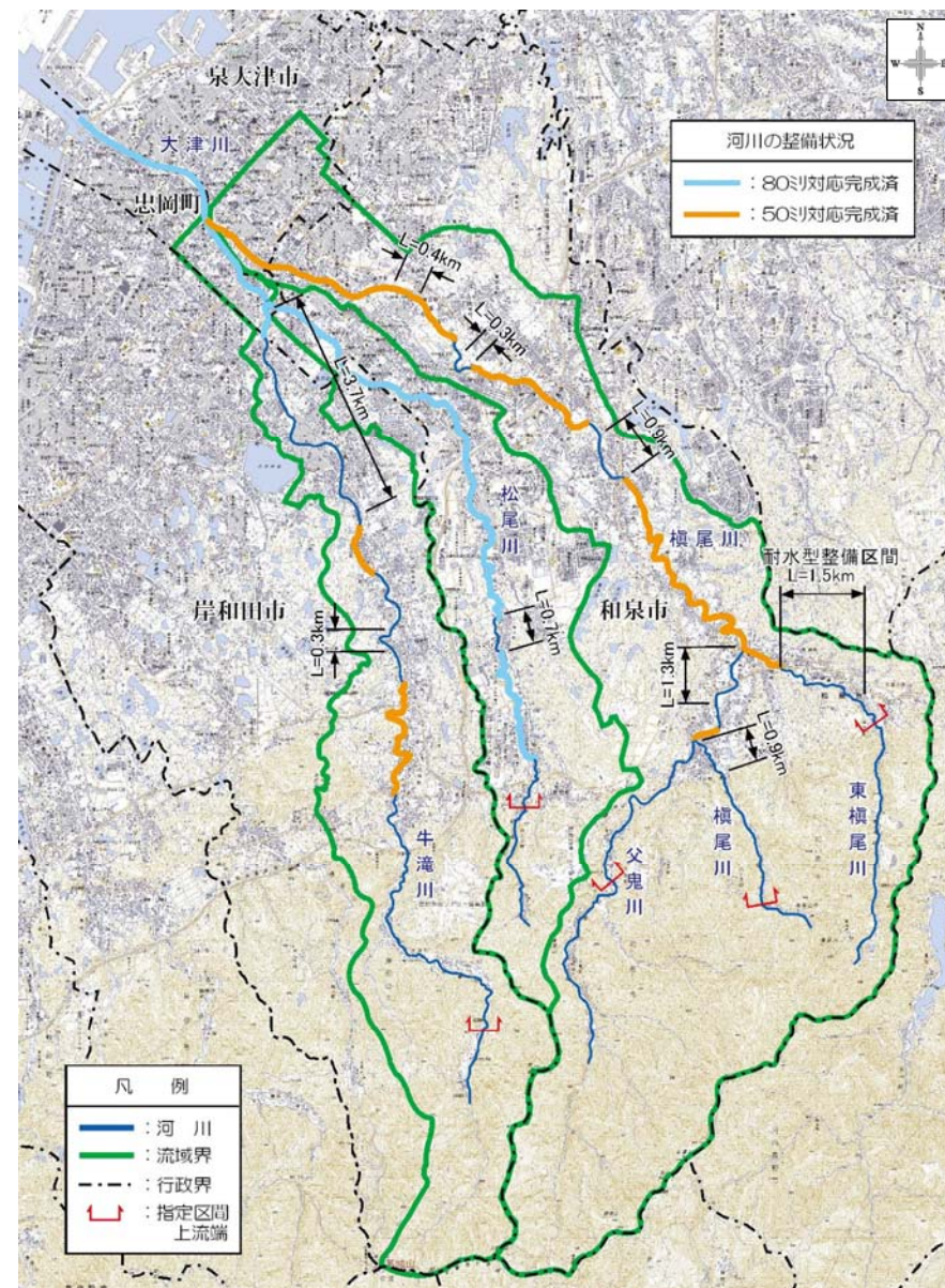
図 2.1.1 整備対象区間平面図（洪水対策）
