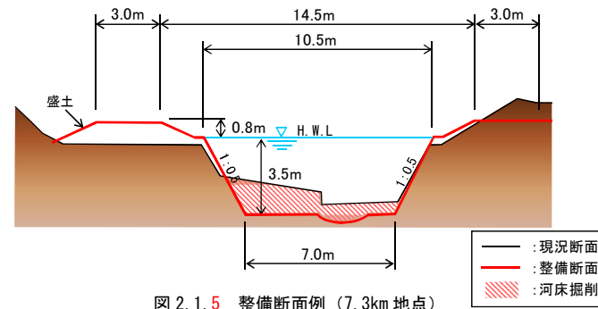
図 2.1.5 整備断面例 (7.3km 地点)
