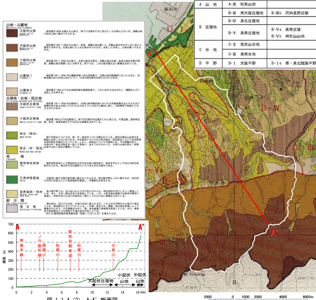
図 1.1.4 (2) A-A' 断面図
