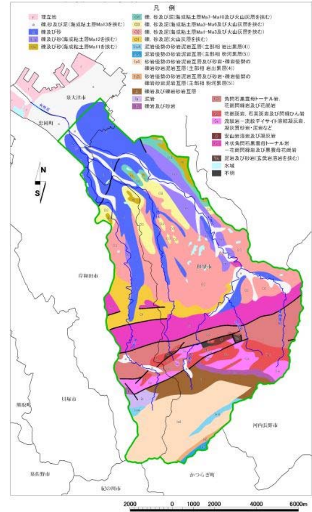
図 1.1.5 大津川流域地質図
