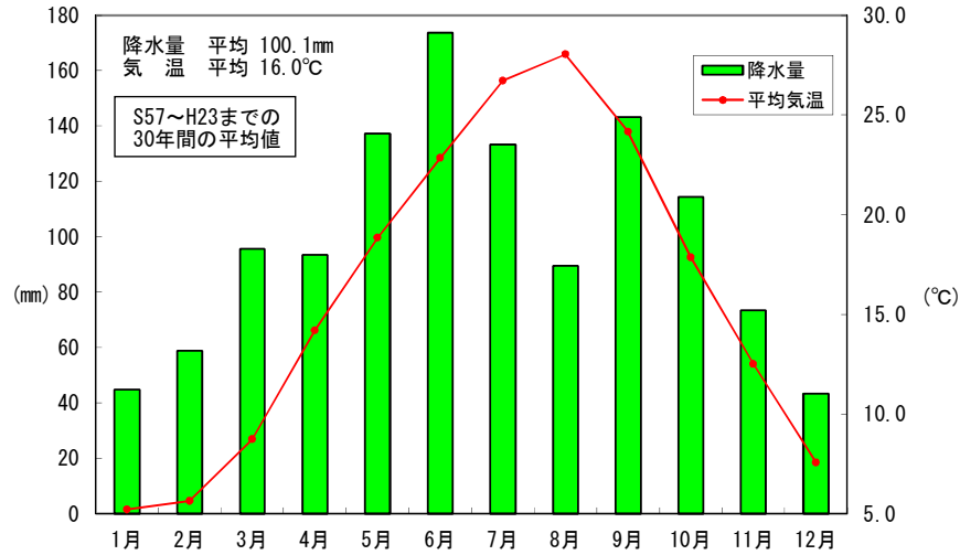
図 1.1.6 月平均降水量・気温（堺観測所）
