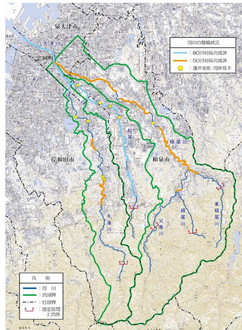
図 1.2.3 大津川水系改修状況図
