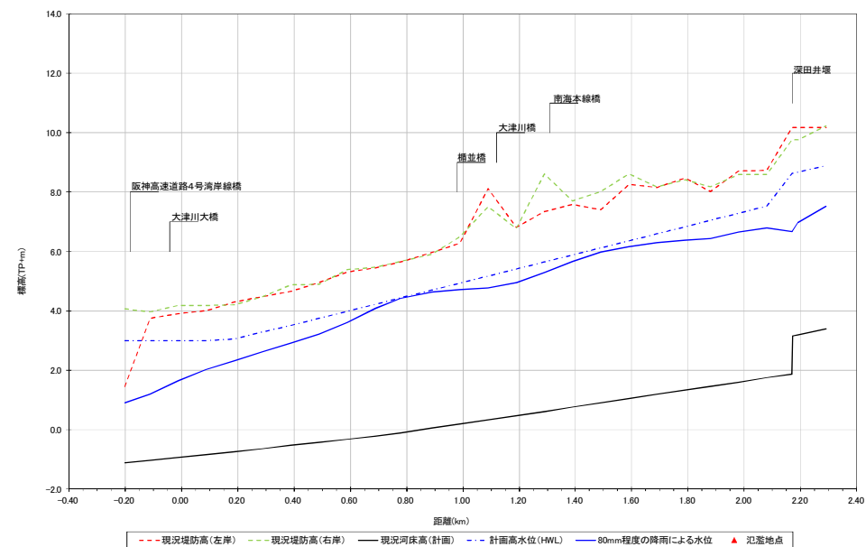
図 1.4.10 大津川水位縦断面図（現況河道：時間雨量 80 ㎥程度）
