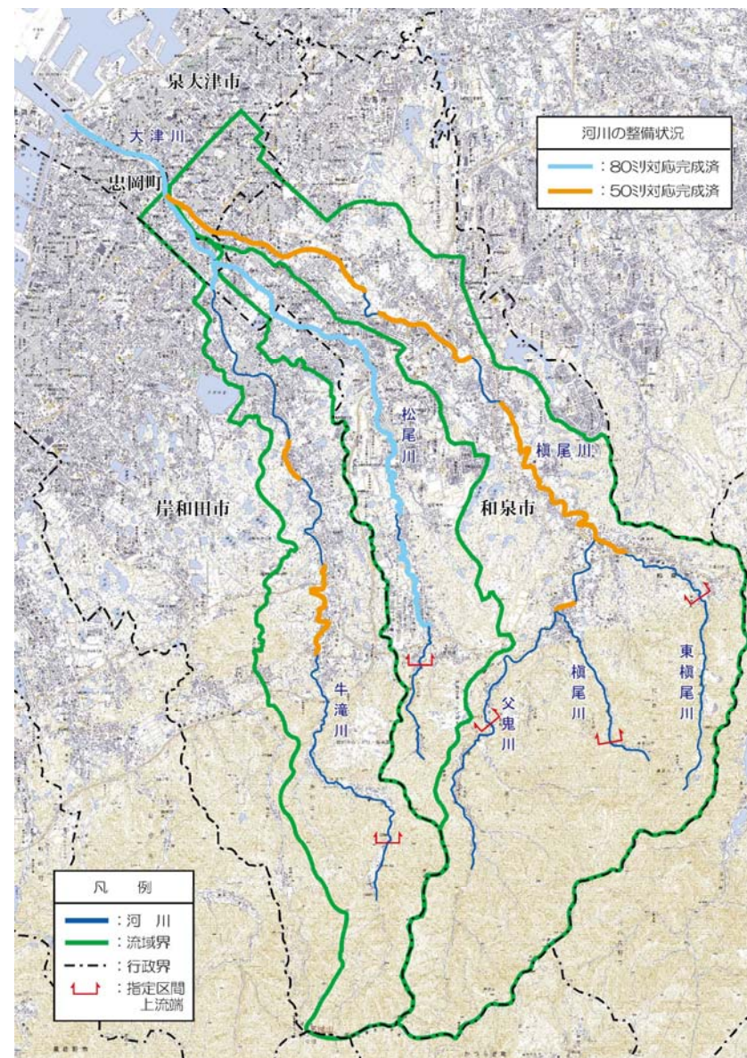
図 1.4.1 治水対策の進捗状況
