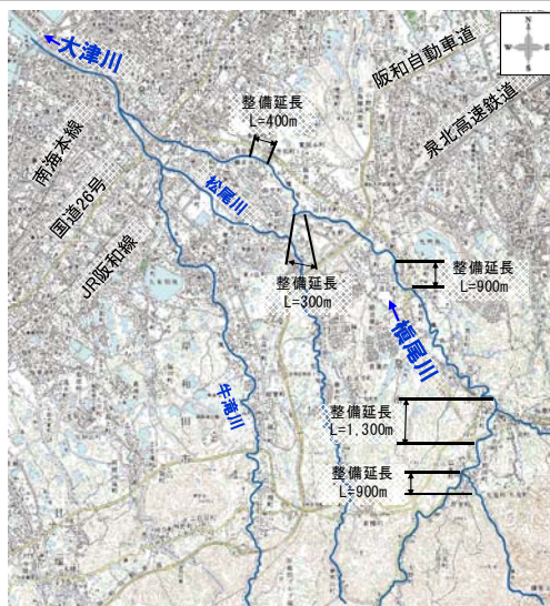
図 2.1.6 整備対象区間平面図
