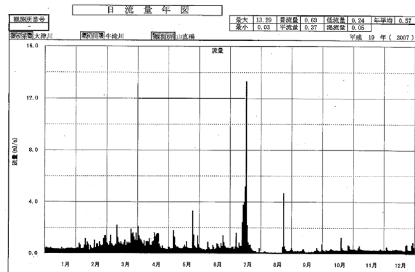
図 1.2.11 日流量年図（牛滝川 山直橋地点 平成19年）
