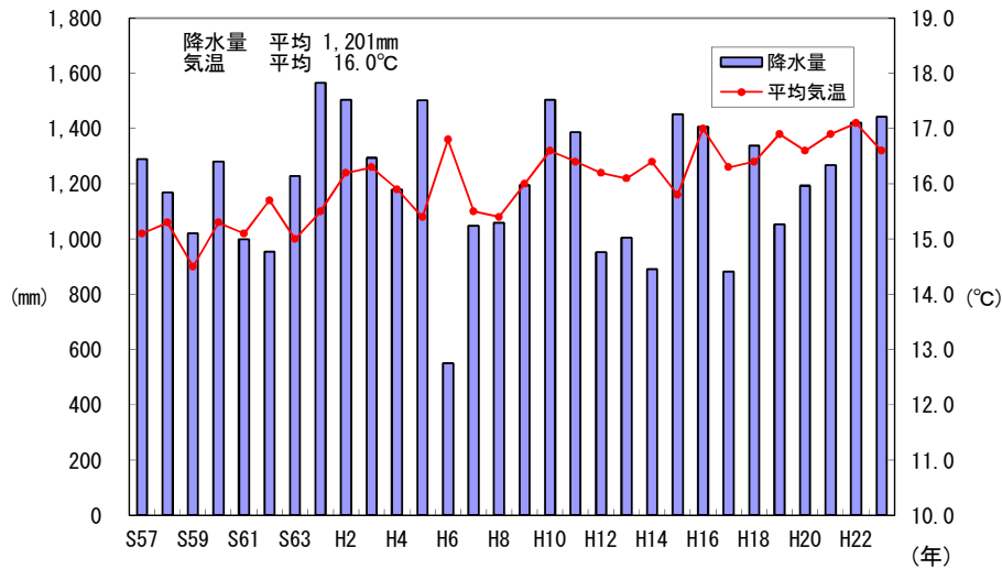
図 1.1.7 年降水量と年平均気温の推移（堺観測所）
