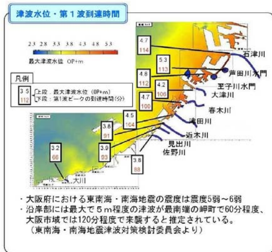
図 1.2.5 津波シミュレーション結果
