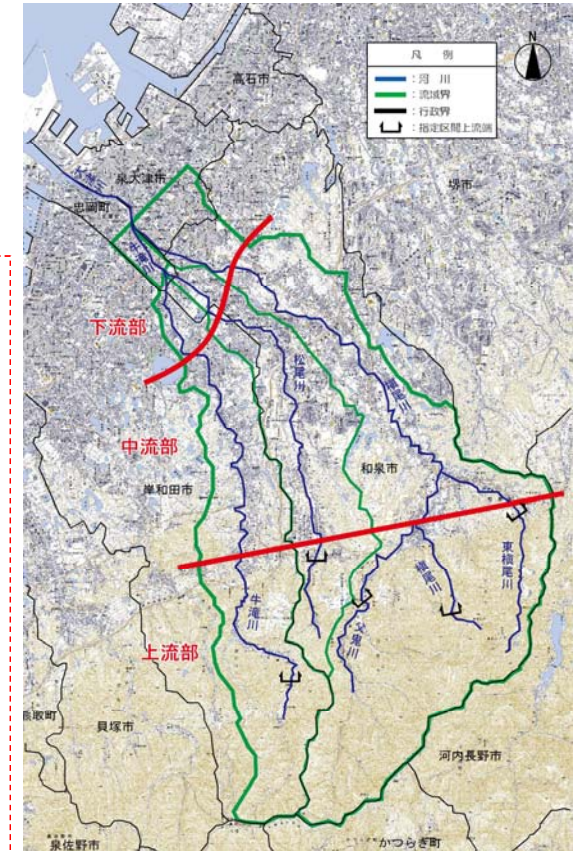
図 1.3.2 大津川水系の流域の区分
