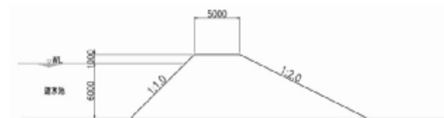
周囲堤の形状
