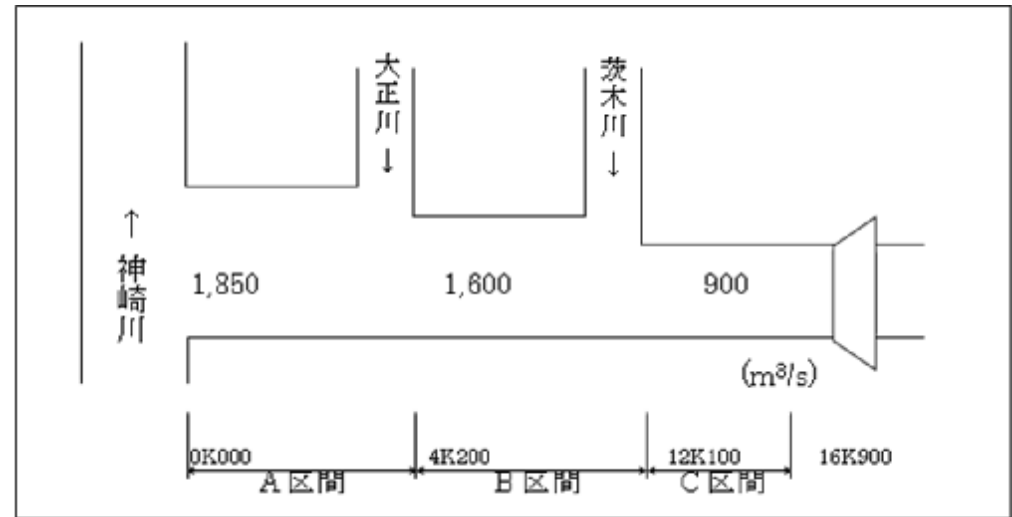
図 4.5.7 安威川基本高水流量
