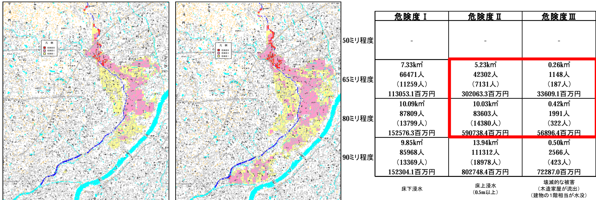
図 4.1.3(1) 現況河道に65mm/h程度 (1/30) の降雨が発生した場合の氾濫解析結果
