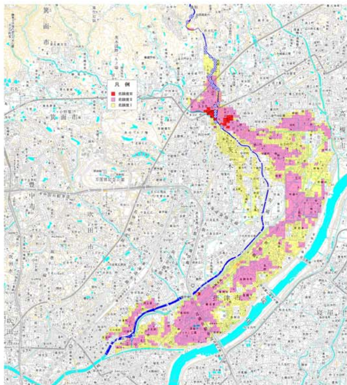
<破堤地点を部分改修した後に80ミ程度の雨が降った場合（1回目）>
