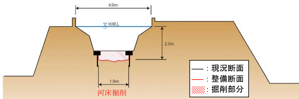
図-2.8 整備断面例 (0.9 km 付近)
