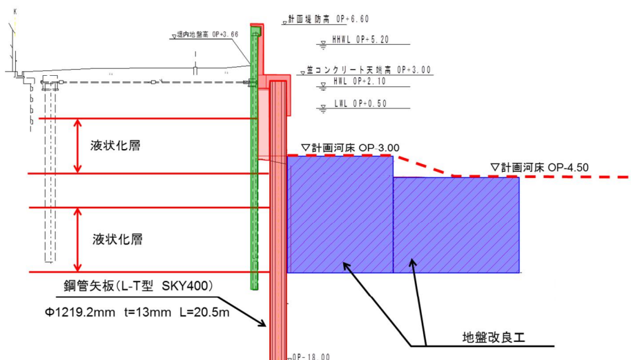
図-2.2 防潮堤耐震補強の標準断面
