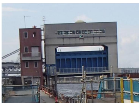
図-1.23 しょうれんじがわ 正蓮寺川水門
