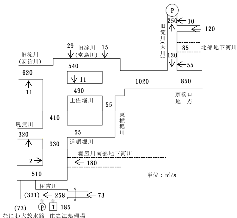
図-1.31 計画高水流量配分図
