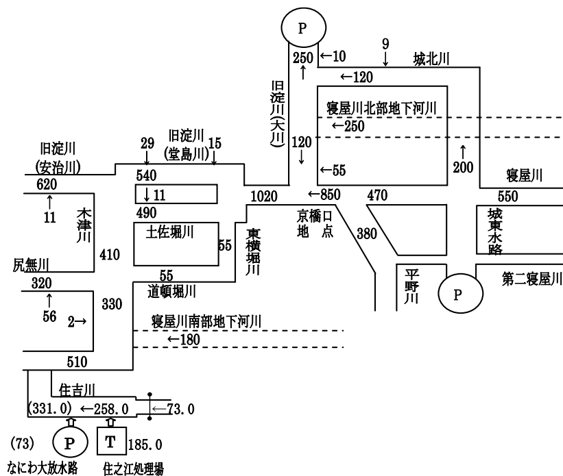
図-1.34 計画高水流量配分図
