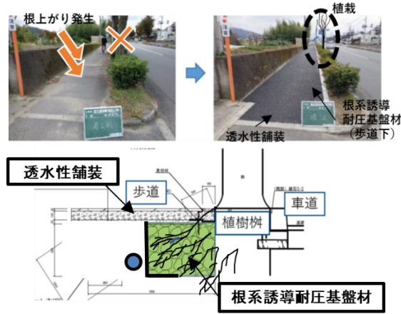
グリーンインフラの取組
