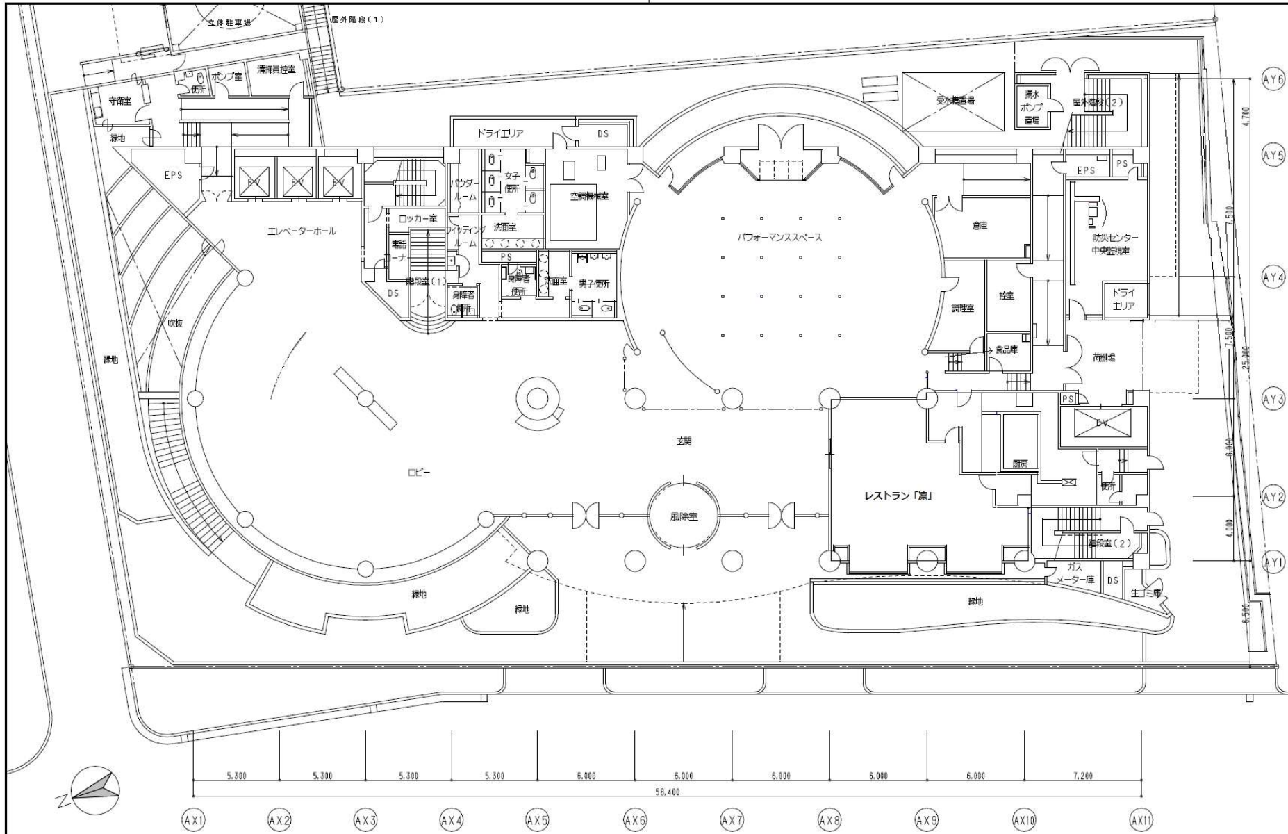
1階平面図 1:200
